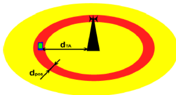
Obrázek 4: Technika TA [10]
