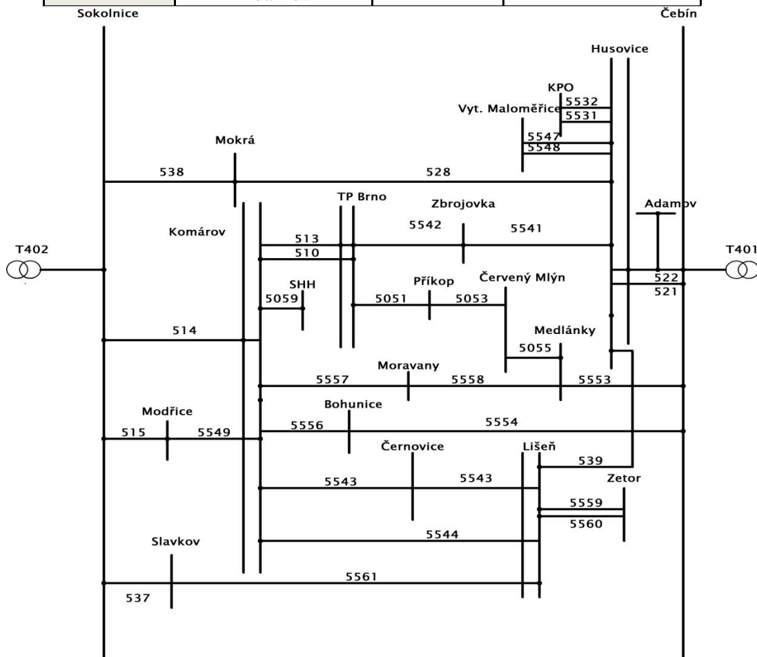
Obr. 6.1 Schéma analyzované sítě (upraveno E.ON)
