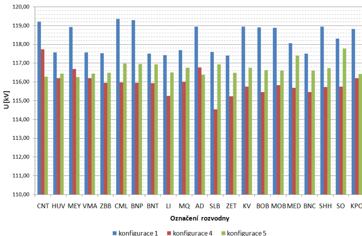
Obr. 9.3 Napěťové poměry v rozvodnách při konfiguracích 1, 4 a 5
