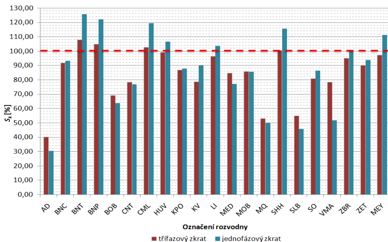
Obr. 10.2 Graf procentního zatížení rozveden zkratovým výkonem při konfiguraci 2
