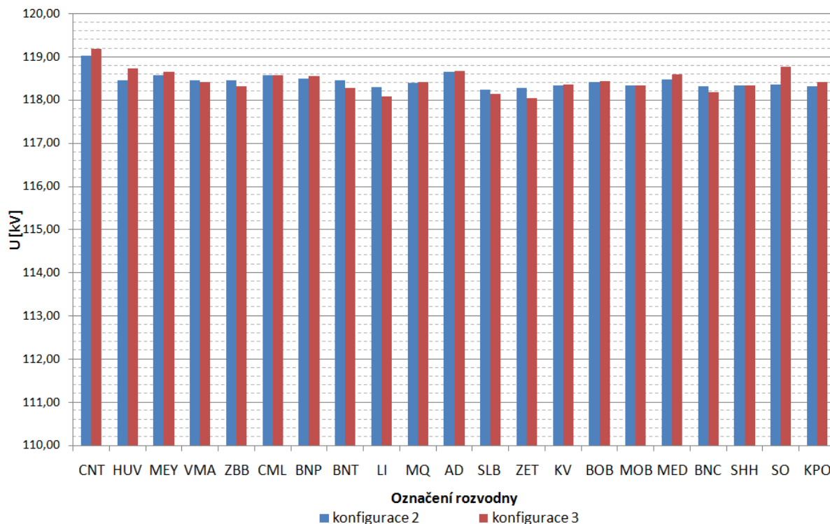
Obr. 9.1 Graf napěťových poměrů v rozvodnách při konfiguracích 2 a 3
