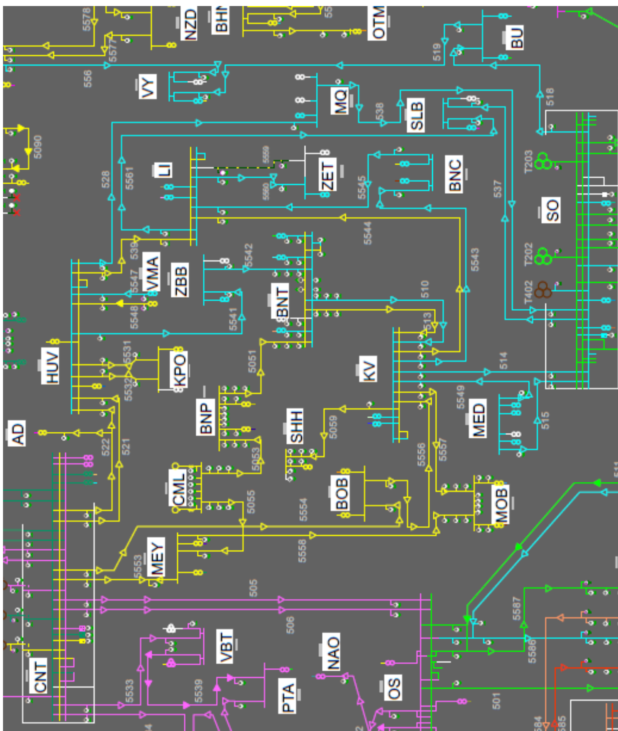
Obr. 0.1 Schéma DS sítě 110 kV základní zapojení – konfigurace 1
