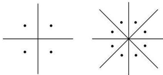
Obr. 4 Degenerované Voroného diagramy
