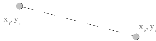
Obr. 3 Spojnice dvou bodů v Euklidovské metrice
