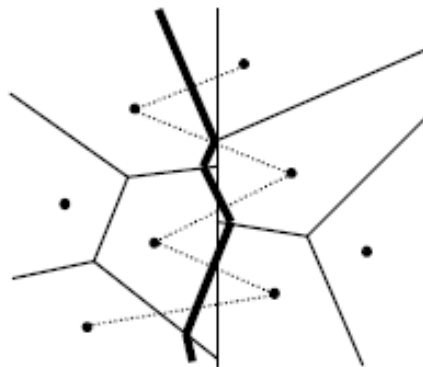
Obr. 12 Propojení dvou podmnožin ve výsledný diagram
