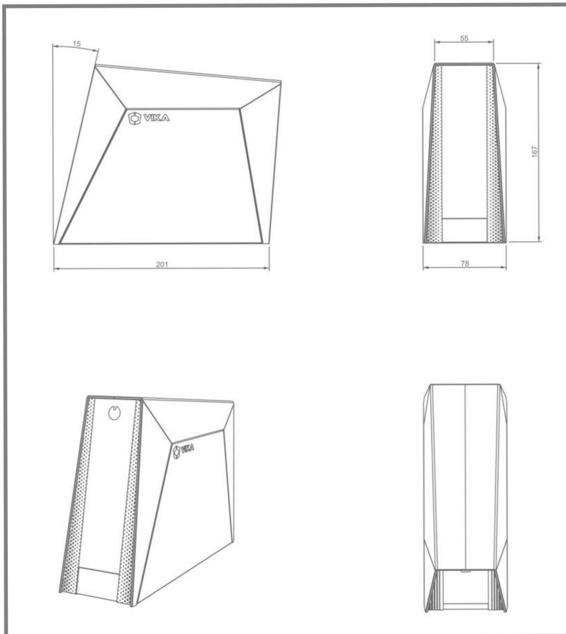
Obr. 23 Vnější rozměry
