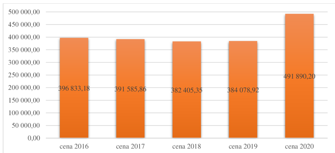
Graf č. 6 Náklady vynaložené na nakladanie s odpadmi v rokoch 2016–2020
