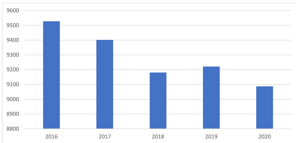
Graf č. 2 Celkové množstvo vyprodukovaného odpadu (v tonách) v podniku „ABC“ v rokoch 2016–2020
