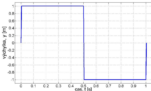
Obr. 1.4: Haarova vlnka
