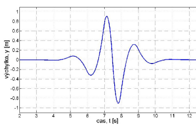
Obr. 1.13: Biortogonální spline 3.3 vlnka
