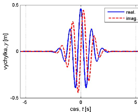
Obr. 1.9: Morletova vlnka
