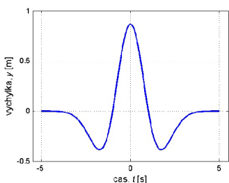
Obr. 1.12: Vlnka Mexican hat
