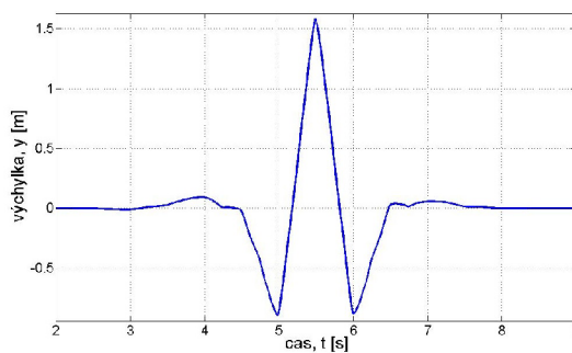
Obr. 1.7: Coiflet 2. řádu
