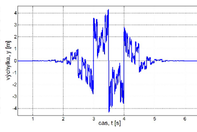
Obr. 1.14: Reverzní biortogonální spline 3.7 vlnka
