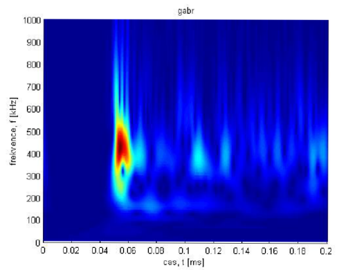
Obr. 6.6: Použití Gaborovy vlnky na signál z obr.6.2
