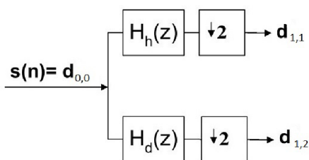
Obr. 1.1: Ukázka rozkladu diskrétní vlnkové transformace
