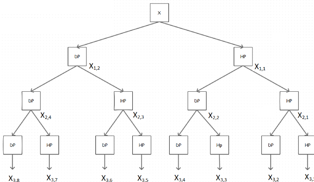
Obr. 7.2: Rozkladový strom WPT použitý při analýze
