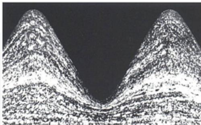
Obrázek č. 2: Výbrus tvářeného závitu vyrobeného válcováním se zřetelnými zpevněnými vnitřními vlákny materiálu (24, s. 58)
