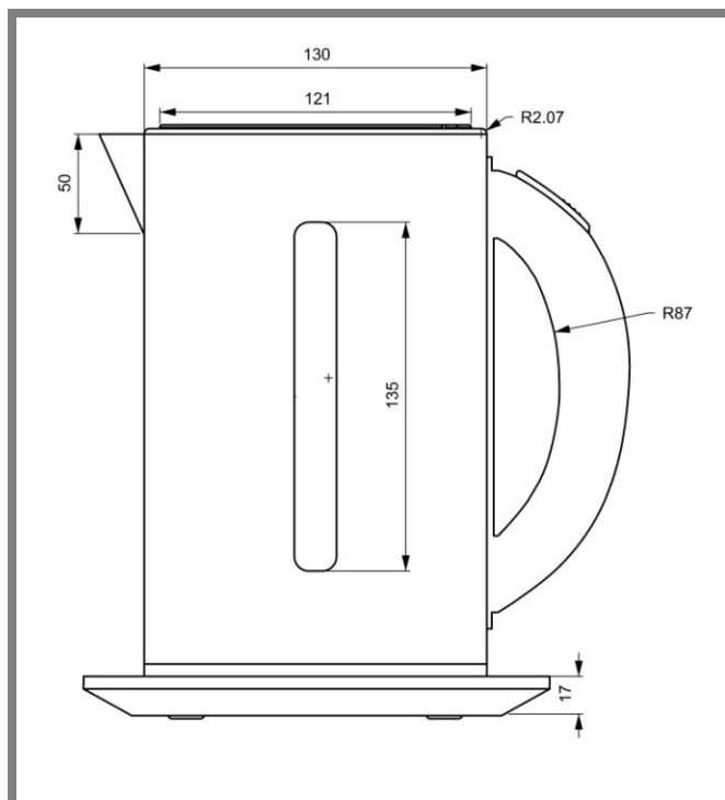
Obr. 5-21 Rozměrové schéma I.
