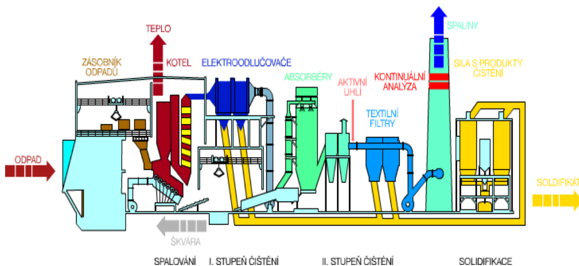
Obr. 4.2 Schéma zařízení spalovny SAKO Brno [29]
