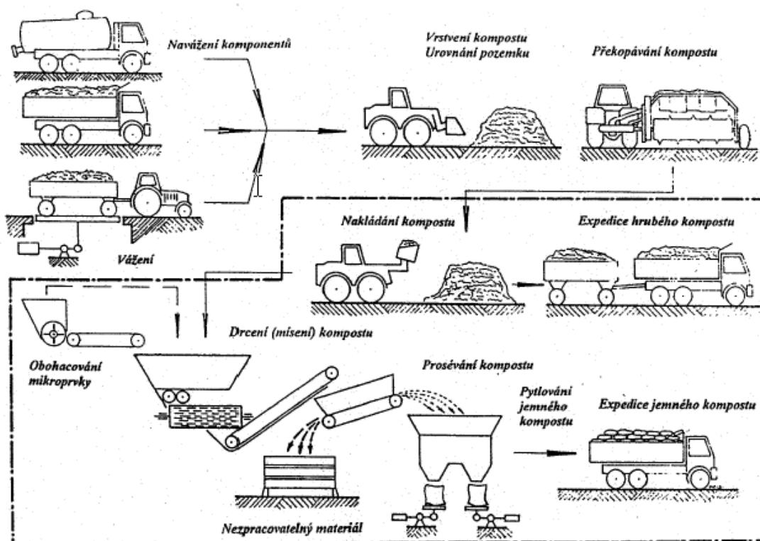
Obr. 4.5 Schéma kompostovací linky [40]
