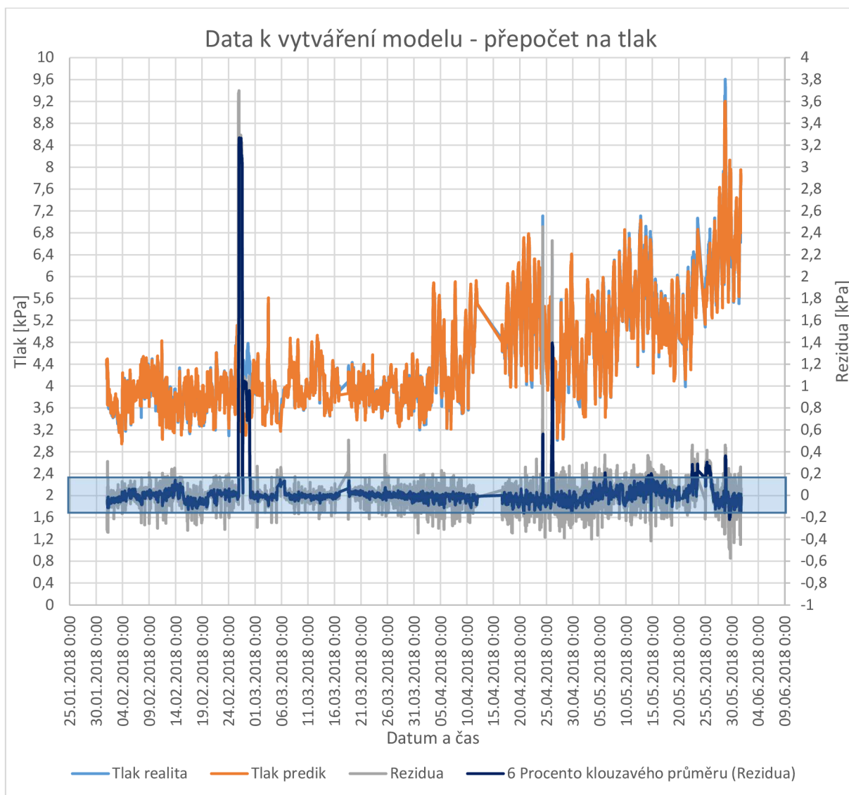
Obr. 29 Graf průběhu hodnot pro modelová data (přepočtená teploty na tlak)
