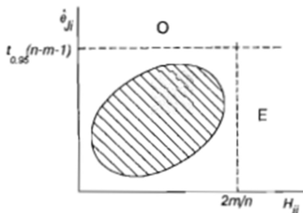
Obr. 13 Williamsův graf [22]
