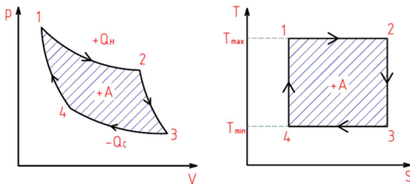
Obr. 2 Carnotův cyklus v p - V a T - s diagramu [3]
