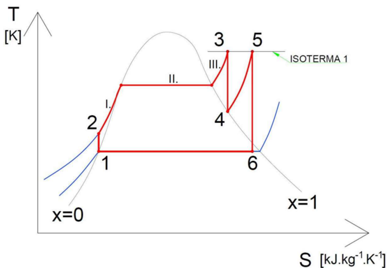
Obr. 9 T-s diagram s přehříváním páry [5]
