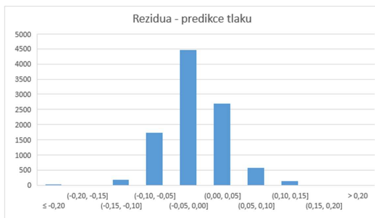
Obr. 23 Histogram reziduí – predikce tlaku
