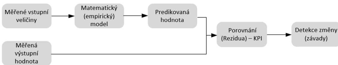
Obr. 32 Princip diagnostiky
