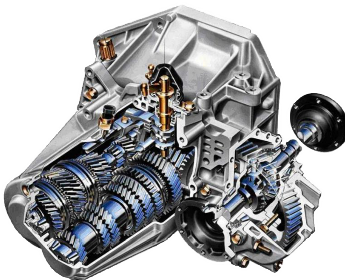
Obrázek 3-13 Převodovka Selespeed [58]
