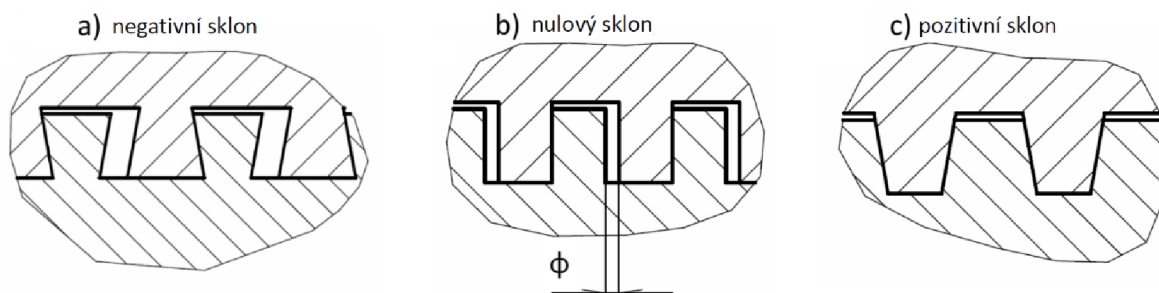
Obrázek 5-48 Základní rozdělení zubových spojek s čelním ozubením dle sklonu boků zubů [107]
