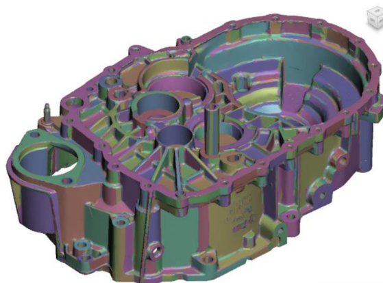
Obrázek 5-14 Výsledek příkazu „Generate face groups“ [zdroj: Autor]
