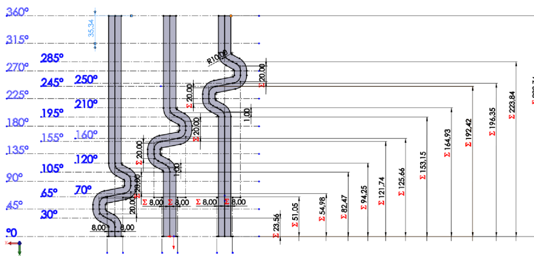
Obrázek 5-43 Náčrt řidicí funkce [zdroj: Autor]
