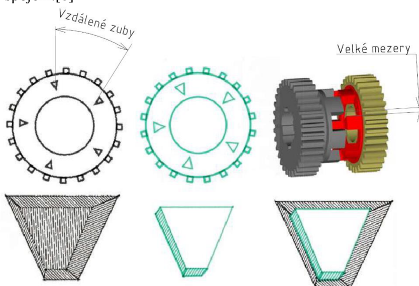
Obrázek 1-3 Zuby zubových spojek [8][9]
