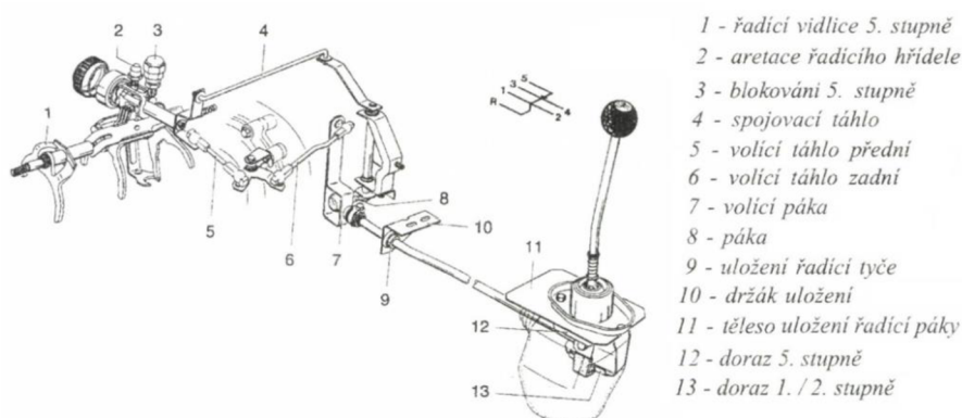
Obrázek 1-11 Řadící ústrojí pětistupňové převodovky VW 020 [2]
