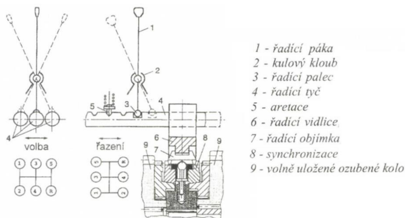
Obrázek 1-10 Přímé řazení pětistupňové převodovky třemi řadícími tyčemi [2]
