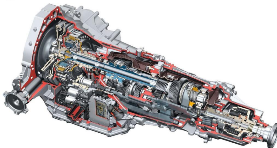
Obrázek 3-24 Sedmistupňová převodovka Audi S-tronic [80]
