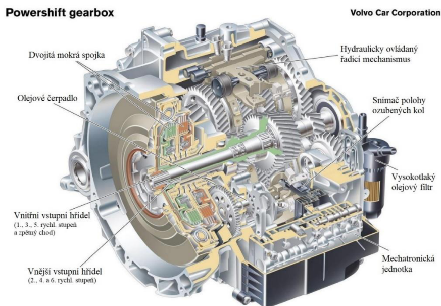
Obrázek 3-23 Převodovka Powershift [78]
