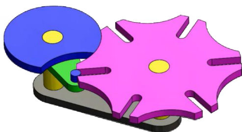
Obrázek 5-39 Maltézský mechanismus [103]
