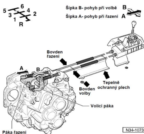
Obrázek 5-38 Řazení převodovky 02Q pomocí bowdenů [102]
