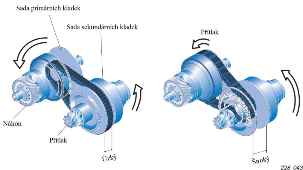
Obrázek 3-15 Převodovka Audi CVT Multitronic 01J [62]
