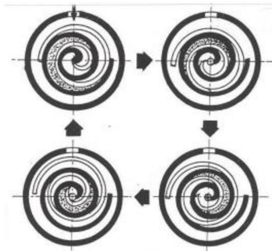
Obr. 12 Princip práce spirálového kompresoru [21]
