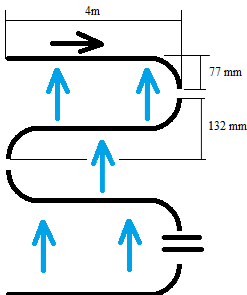
Obr. 19 Schéma varianty s měděnými trubkami \text{Ø}D = 22 \text{ mm}
