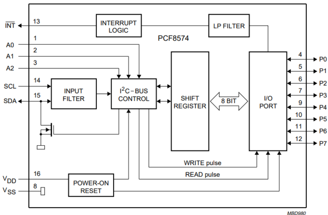
Obrázek 12: Blokové zapojení expandéru [21]
