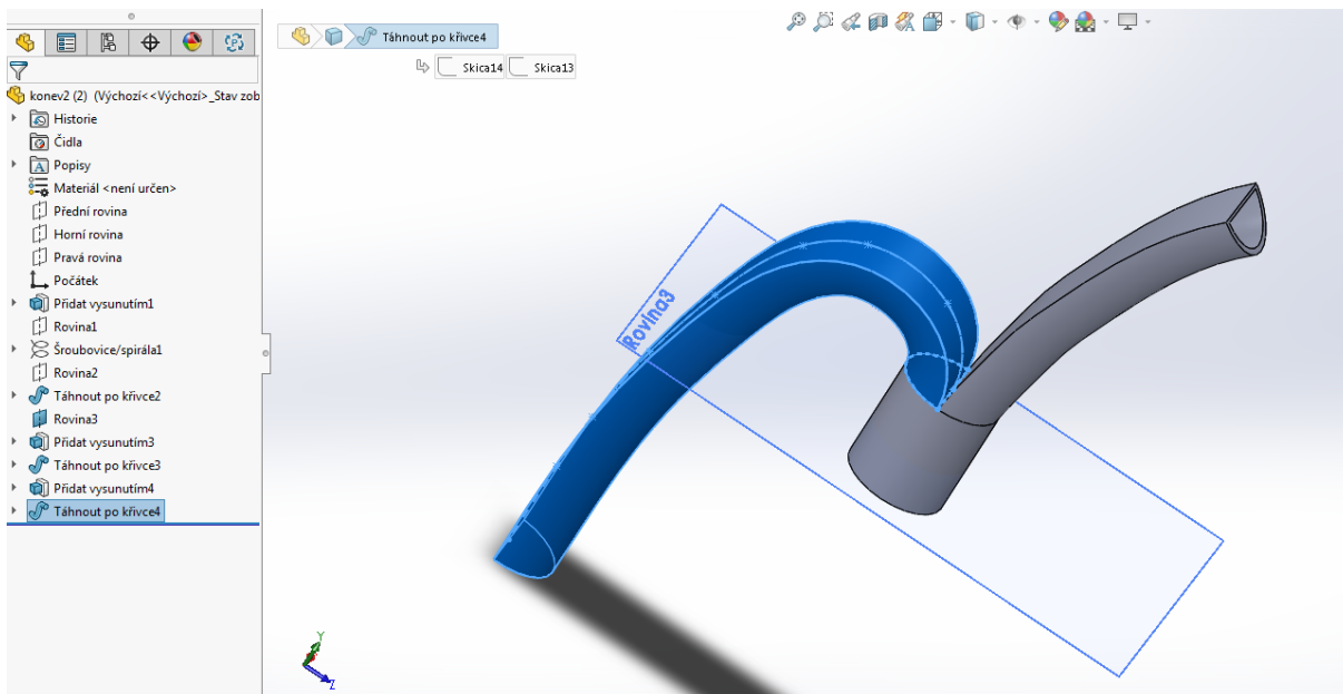
Obr. 14: Konstrukce držadla (7).
