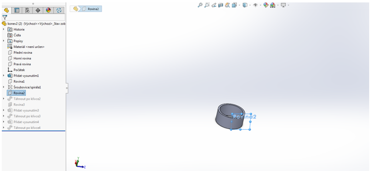
Obr. 8: Vložení roviny 2 (7).
