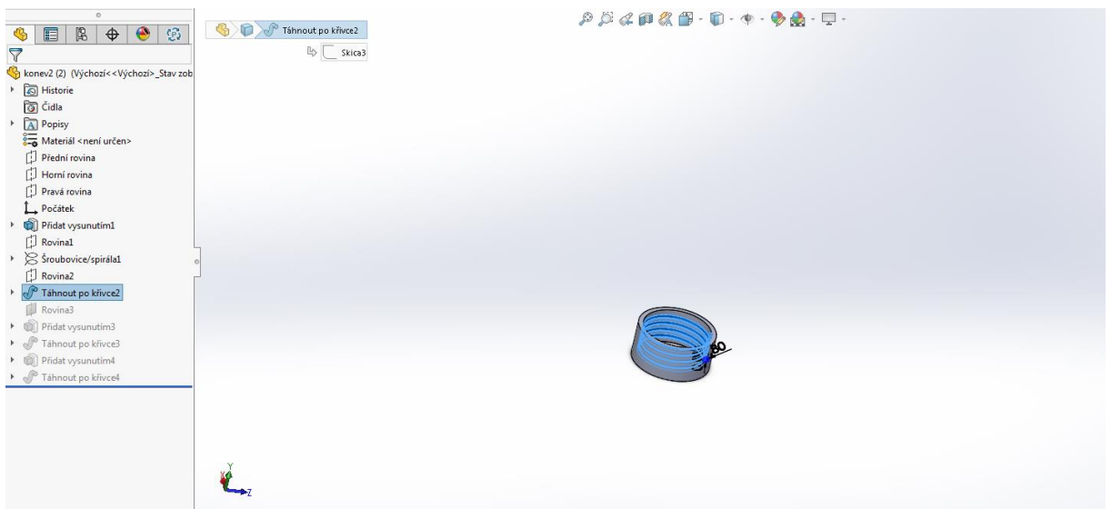
Obr. 9: Vytvoření závitu (7).
