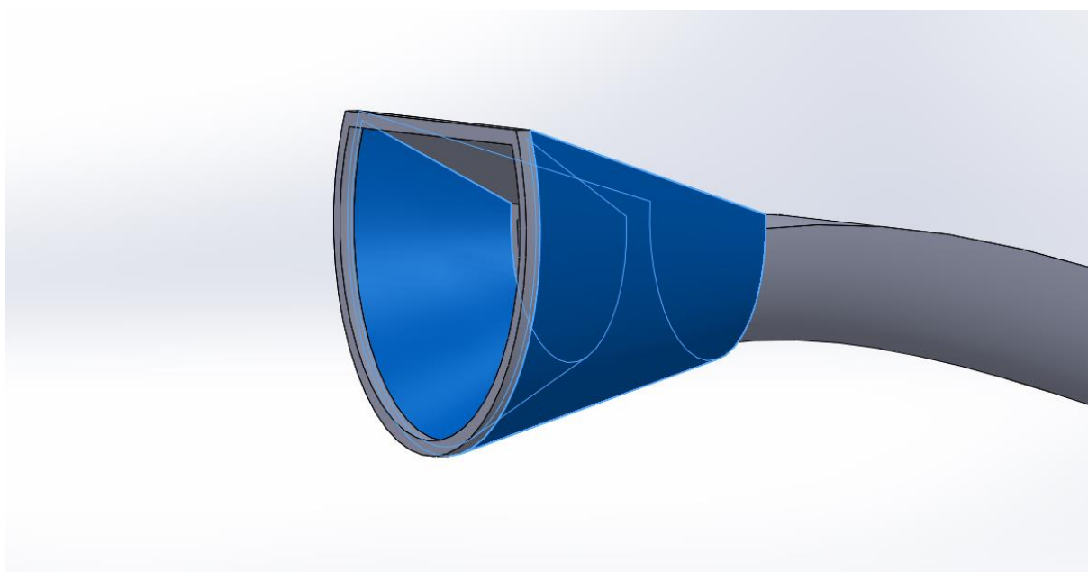
Obr. 22: Spojení profilů 2 (7).
