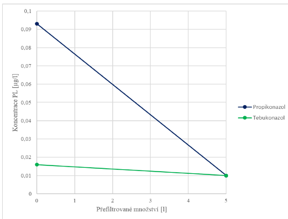
Obr. 7.21 Koncentrace PL po filtraci přes AU Silcarbon K 835 [autor]
