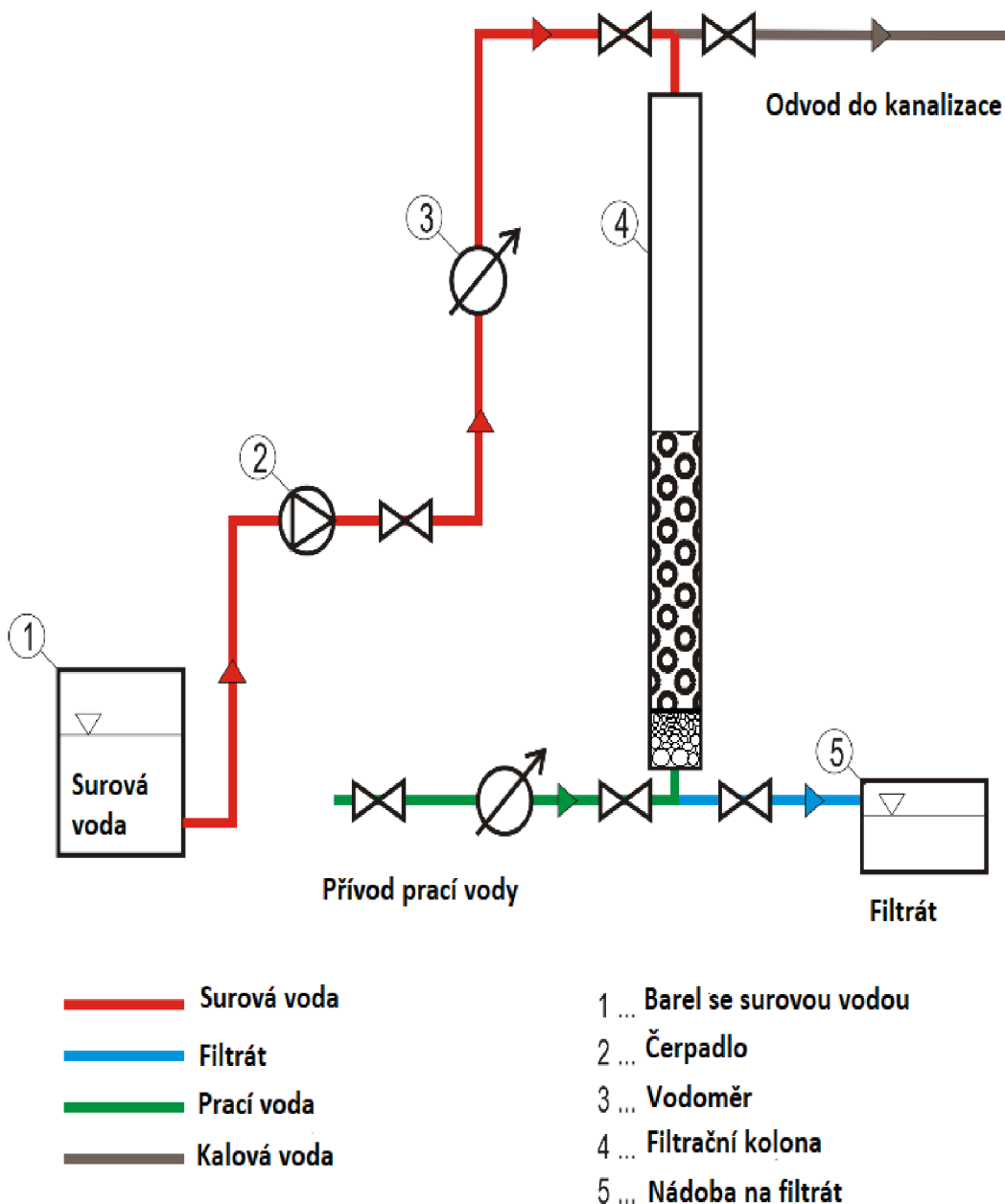
Obr. 7.7 Schéma filtračního zařízení [autor]
