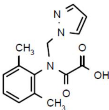
Obr. 7.18 Chemický vzorec Metazachloru OA [52]
