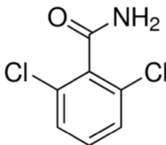
Obr. 7.19 Chemický vzorec BAM [61]
