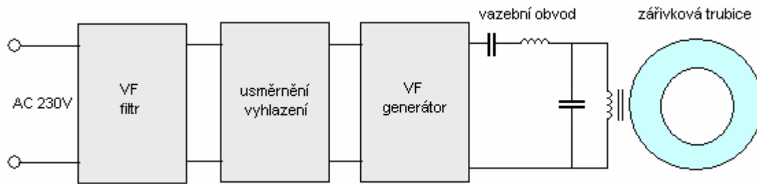
Obr. 3-14 Funkční schéma indukční zářivky
