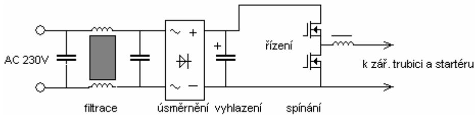
Obr. 3-9 Předřadník kompaktní zářivky bez aktivního filtru
