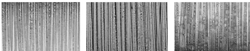
Obrázek 8.10: Vlákna PP výměníku z 6 vrstev a 3 mm mezer v průběhu experimentu s rychlostí 1 m/s a 50 % relativní vlhkost, vertikální poloha (vlevo), 45° (uprostřed), horizontální poloha (vpravo).
