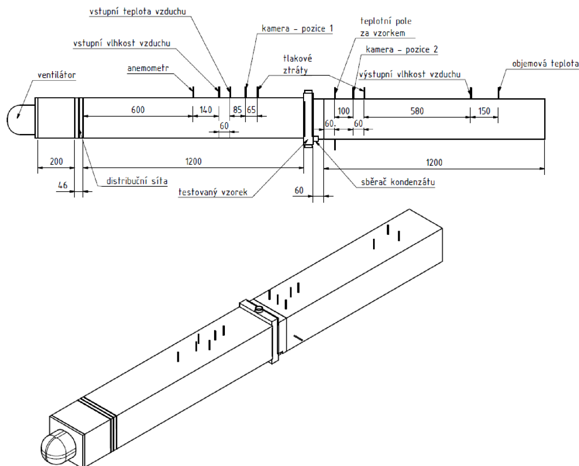
Obrázek 8.2: Schéma větrného tunelu osazeného měřicími sondami.
