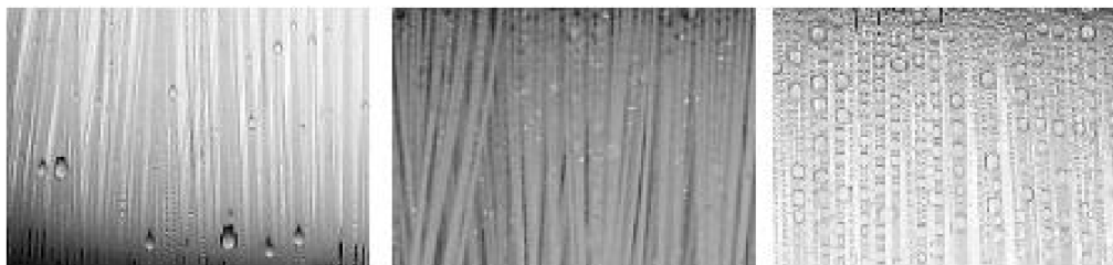
Obrázek 8.9: Vlákna PP výměníku s 6 vrstvami po 8 mm v průběhu experimentu s rychlostí 3 m/s a 50 % relativní vlhkost, vertikální poloha (vlevo), 45° (uprostřed), horizontální poloha (vpravo).
