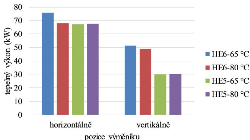
Obrázek 7.14: Tepelný výkon při maximálním průtoku vody ve vláknech, který byl výměník schopen ohřát na požadovanou teplotu (65 °C, 80 °C).
