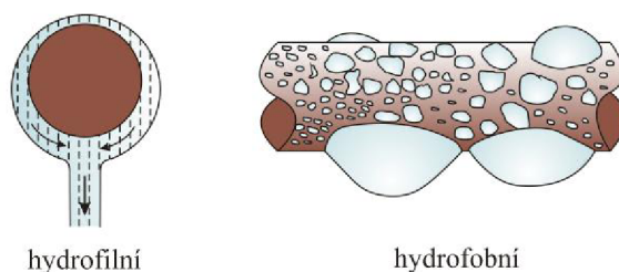
Obrázek 6.3: Kondenzace na povrchu radiálního tělesa a jeho možné stékání. (Upraveno podle [11].)
