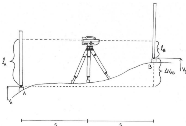
Obrázek 2.5 - Geometrická nivelace ze středu (vlastní)
