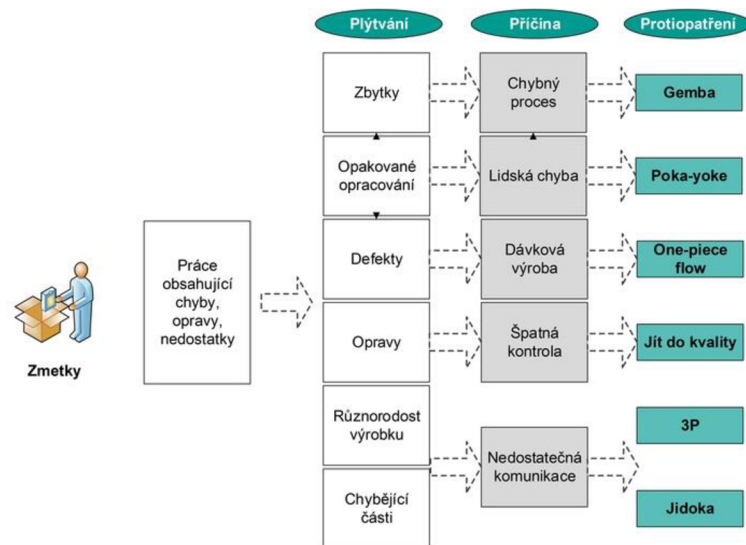
Obrázek 1.5: Tvorba zmetků [16]
