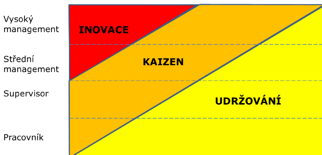
Obrázek 1.7: Kaizen [12]
