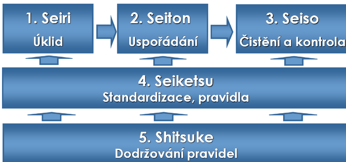
Obrázek 1.10: Metoda 5S
