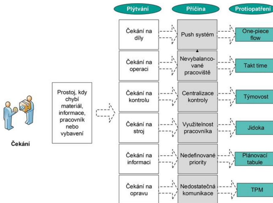
Obrázek 1.2: Čekání [16]
