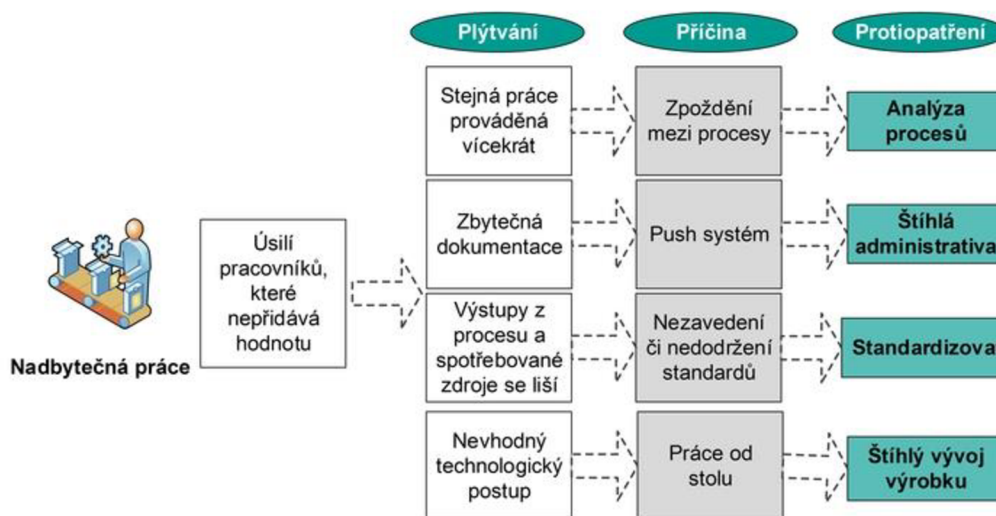
Obrázek 1.4: Nadbytečná produkce [16]
