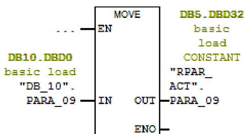
Obrázek 8: Použití bloku Move s opravdovými hodnoty
