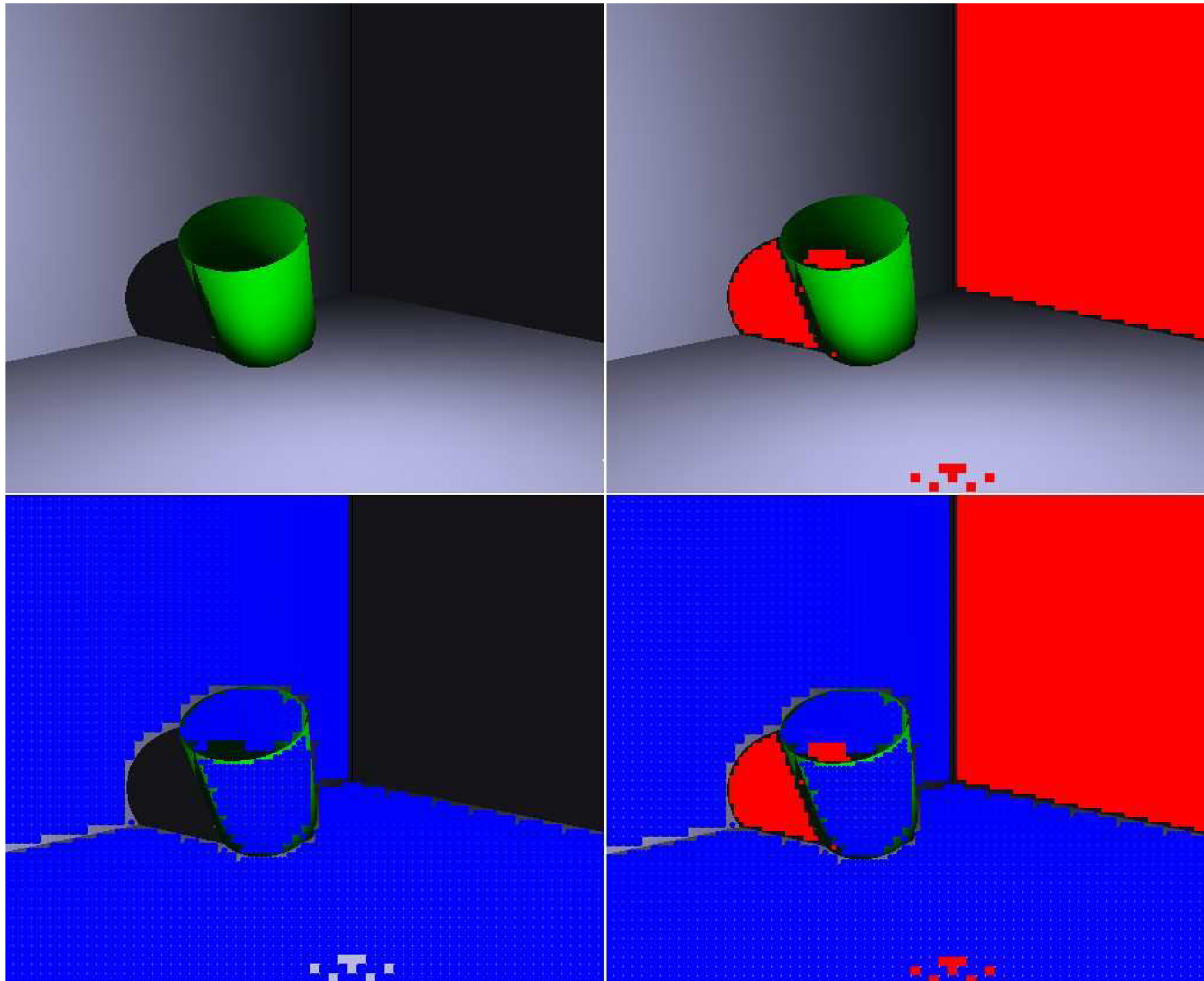
Obrázok 5.1 – Demonstrácia implementovanej techniky adaptívneho podvzorkovania v kombinácii s bilineárnou interpoláciou. Červená predstavuje body vyfarbované na základe totožnosti farby, modrá predstavuje body interpolované.
