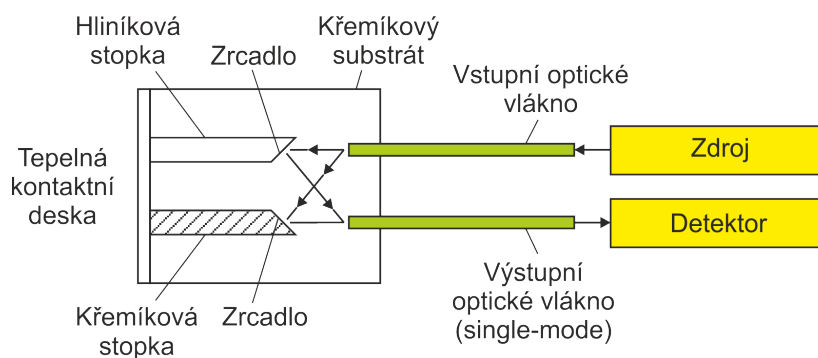
Obr. 5.2: Reflexní optický snímač teploty využívající diferenciální teplotní roztažnost.
