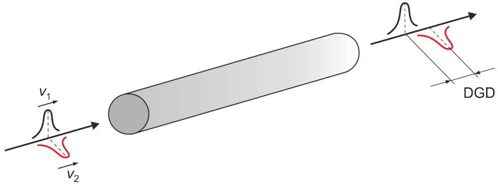
Obr. 1.3: Diferenciální skupinové zpoždění [9].
