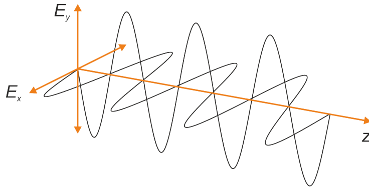
Obr. 1.1: Grafické znázornění elektromagnetického vlnění [1].
