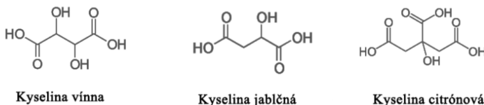
Obrázok 1: Štruktúrne vzorce kyseliny jablčnej, vínnej a citrónovej [29]
