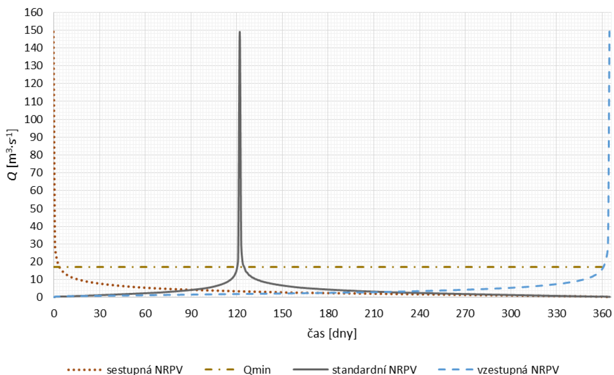
Obr. 6.17 Extrapolované průtoky NRPV (3 varianty) a průtoku Q_{min}
