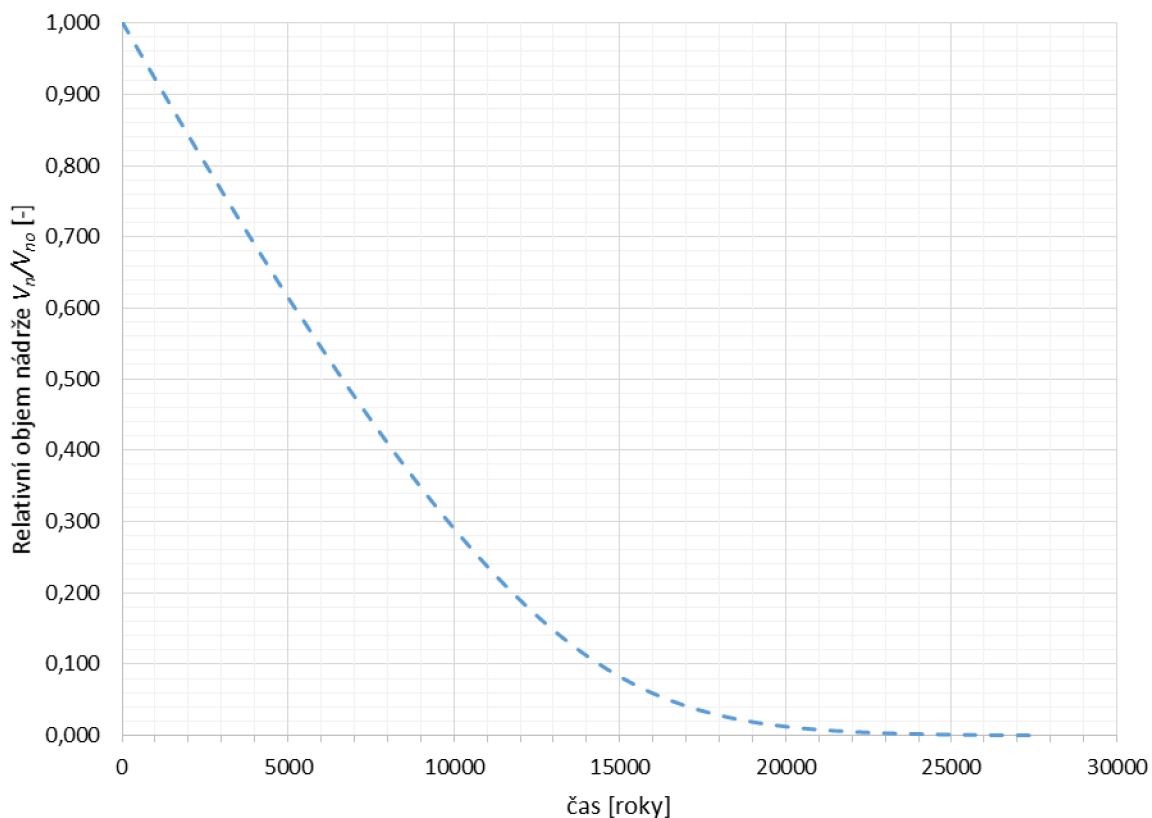
Obr. 8.2 Vyhodnocení životnosti nádrže - varianta SUP
