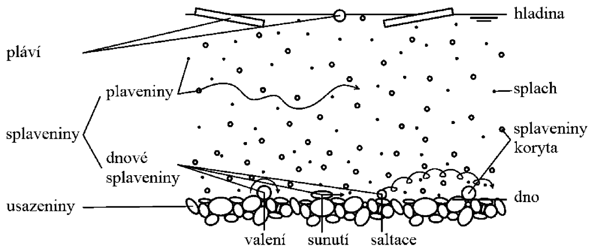
Obr. 3.1 Dělení částic v korytě toku dle jejich pohybu v proudu [4]
