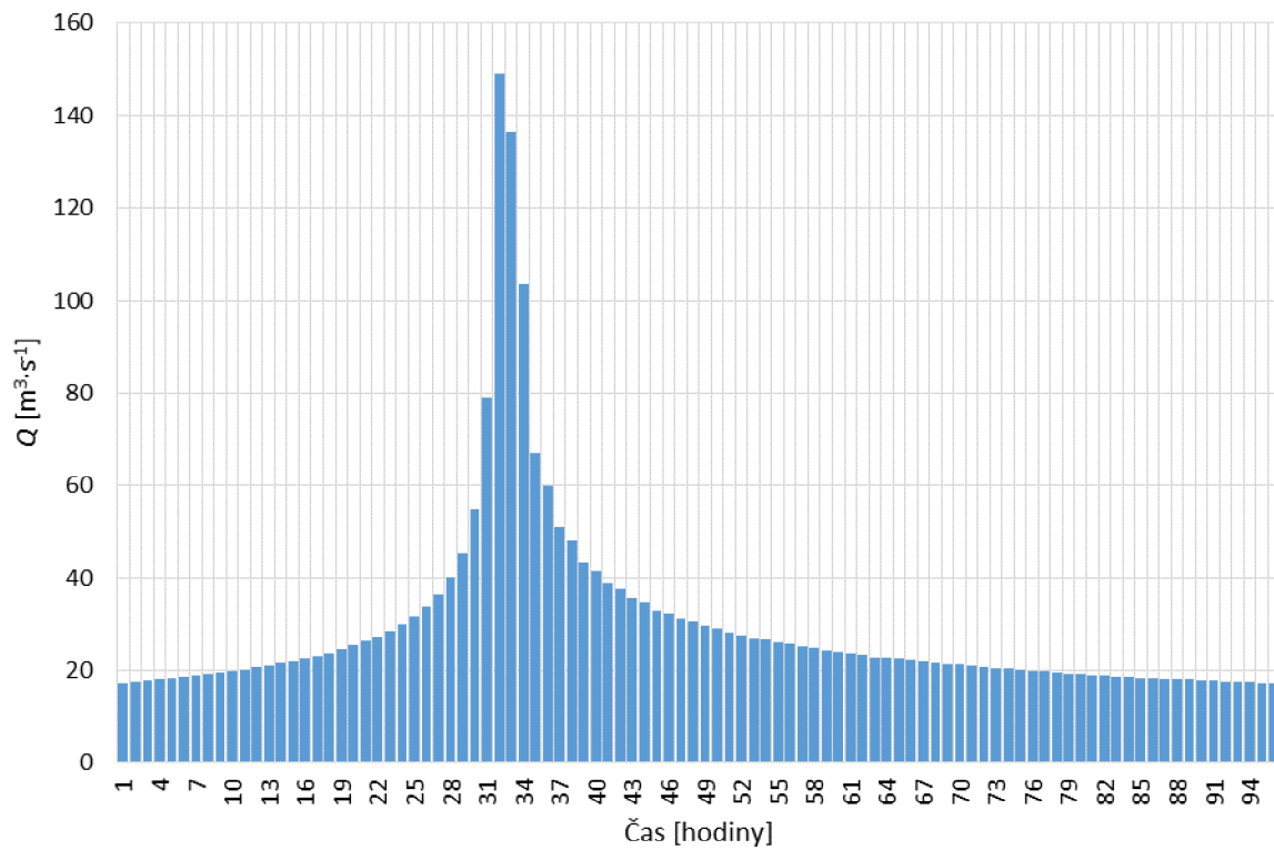
Obr. 6.18 Standardní NRPV
