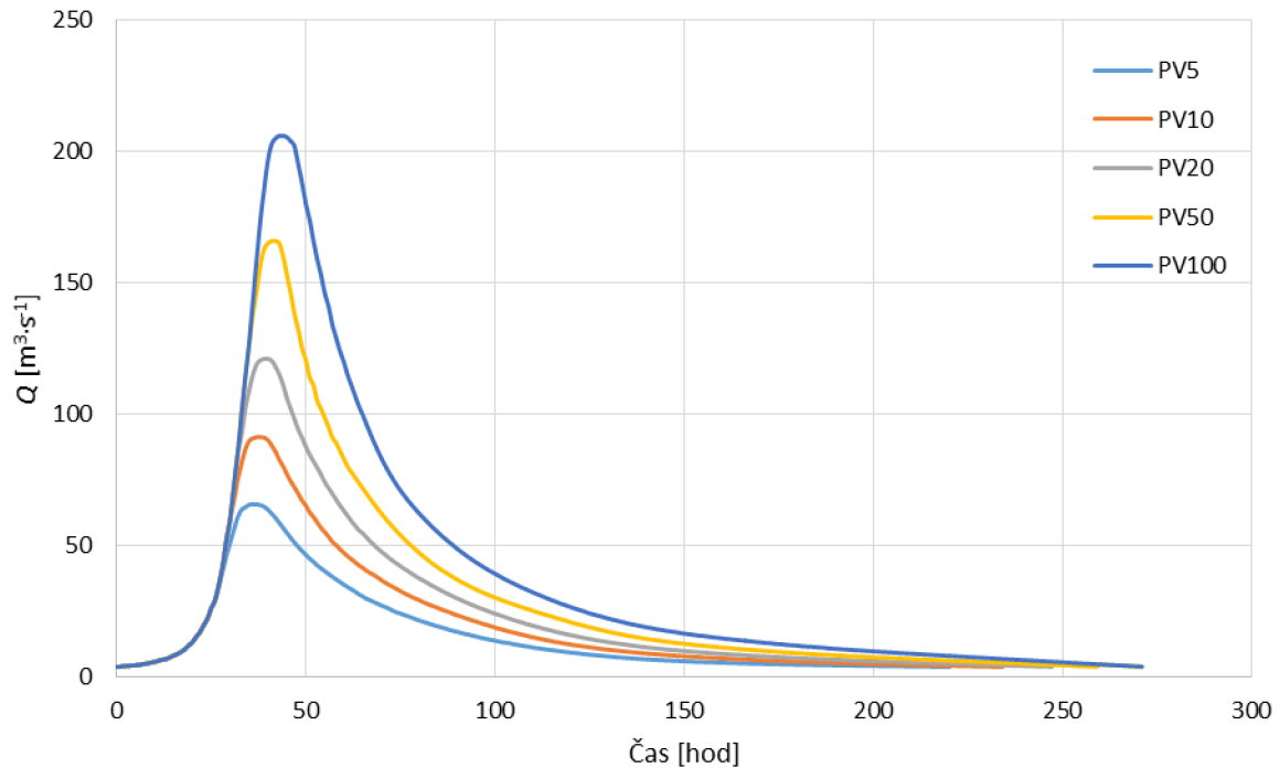
Obr. 6.8 Povodňové vlny [7]
