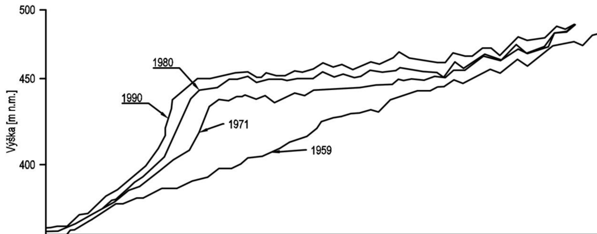
Obr. 4.7 Podélný profil nádrže Bhakra v Indii (podélné staničení nebylo součástí obrázku) [3]
