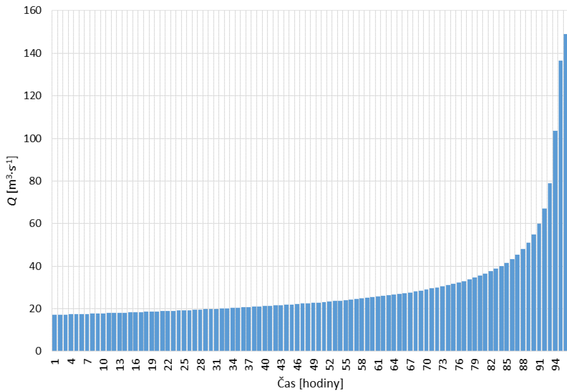
Obr. 6.20 Vzestupná NRPV
