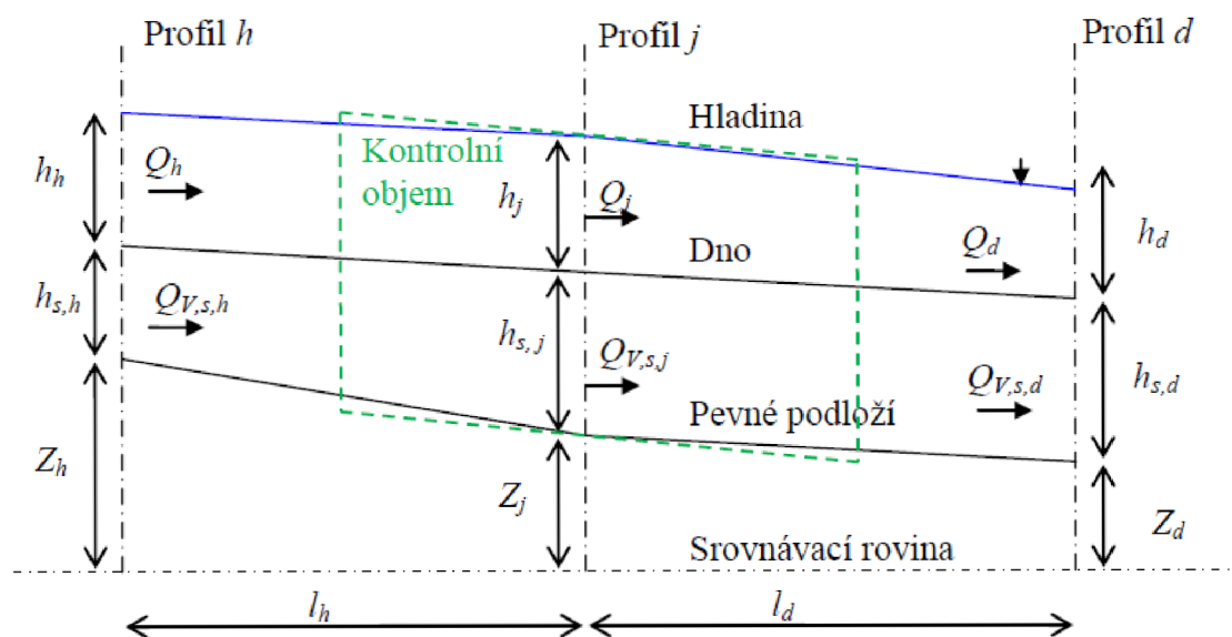
Obr. 3.8 Schéma pro výpočet spojitosti splavenin [7]
