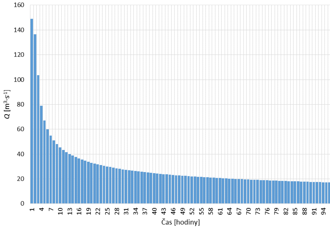
Obr. 6.19 Sestupná NRPV
