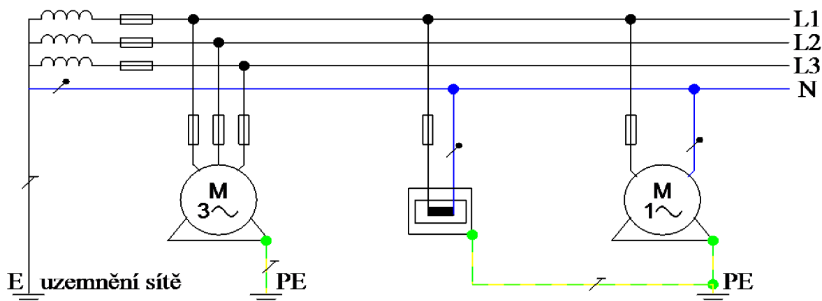
Obr. 2-3 Síť TT
