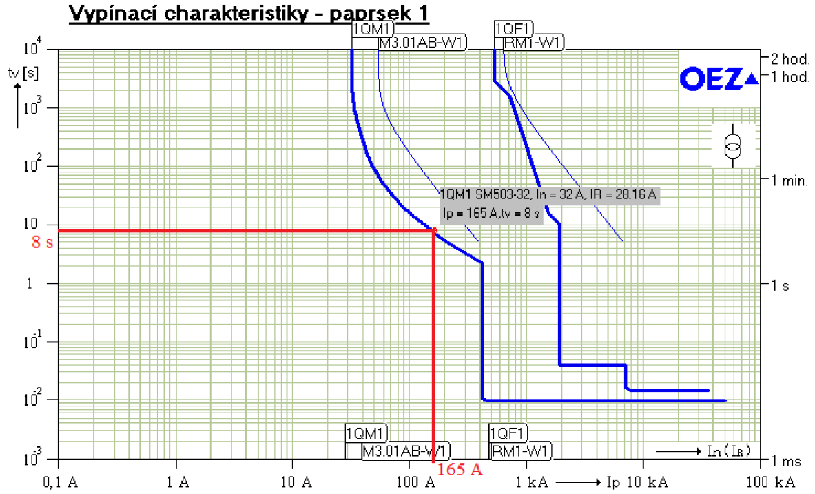
Obr. 5-4 Vypínací charakteristiky - paprsek 1 z programu Sichr.
