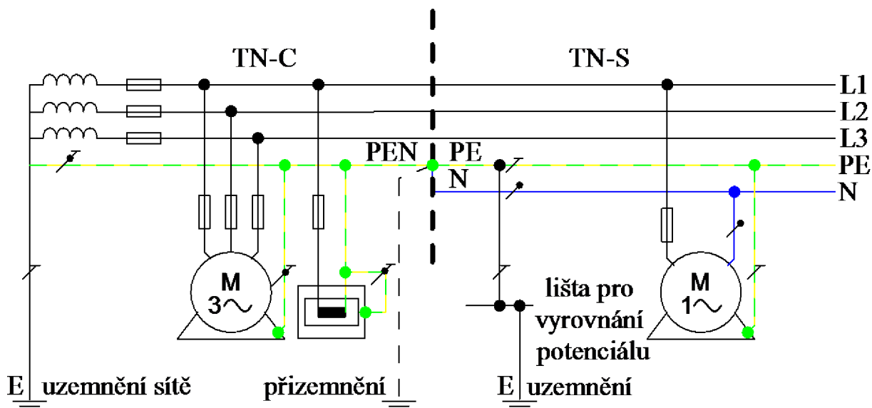
Obr. 2-2 Síť TN-C-S[1].
