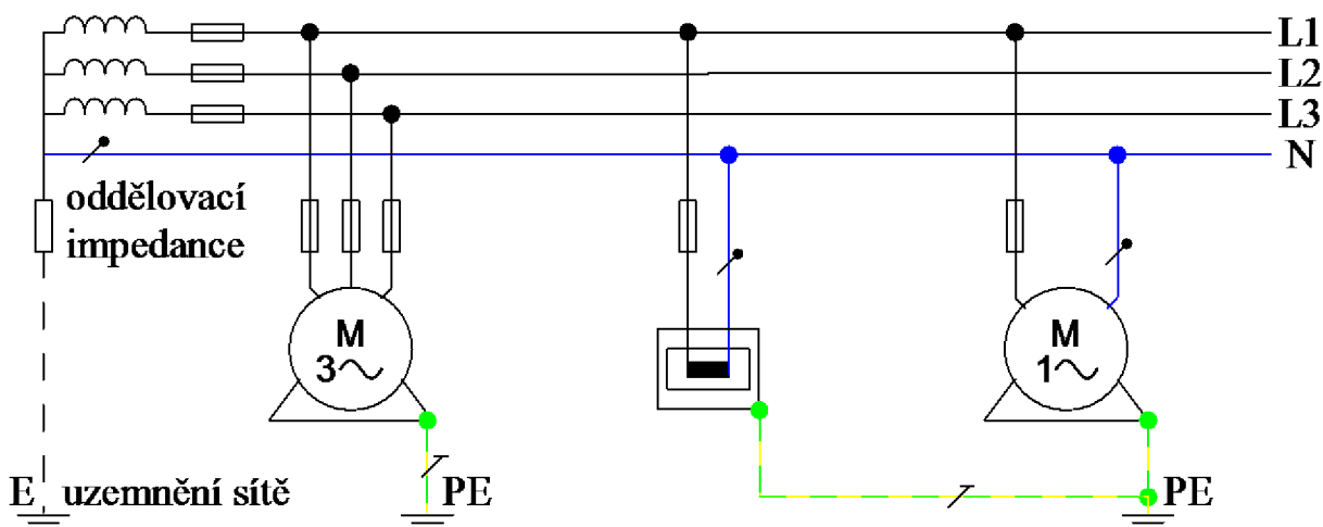
Obr. 2-4 Síť IT
