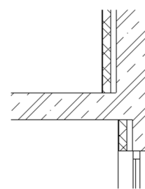
Obr. 67 Začištěný spoj stěn
