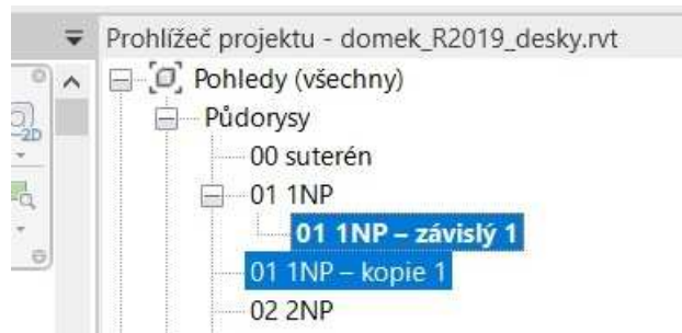
Obr. 17 Hierarchie pohledů
