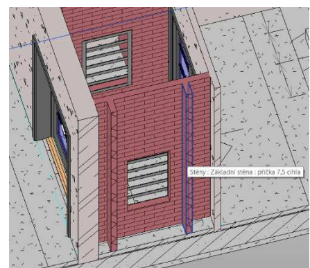
Obr. 62 Ukázka krytu větrací šachty v BP
