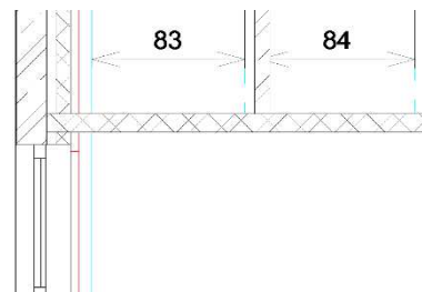
Obr. 68 Problematický spoj na styku příčky a obvodové stěny
