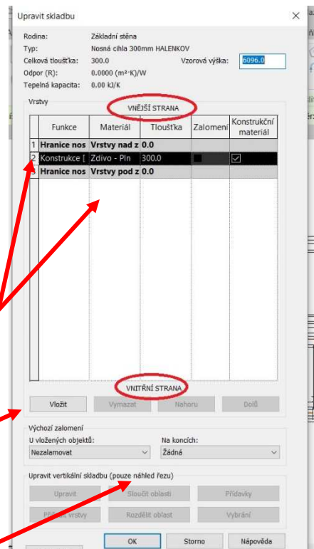
Obr. 47 Upravit skladbu
