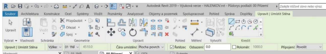
Obr. 41 Karta Upravit
