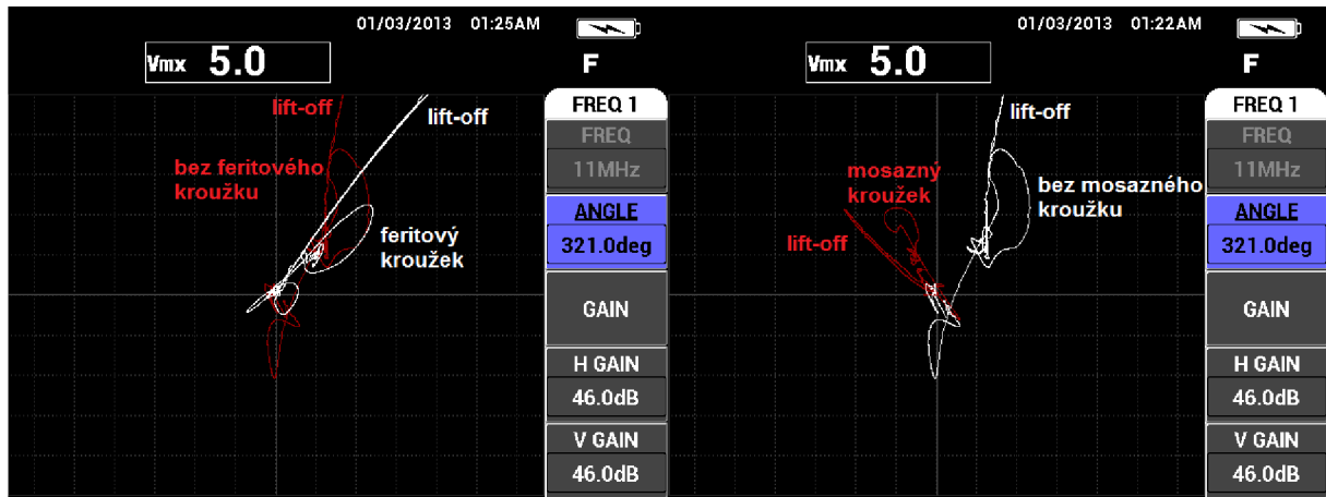
Obr. 7.32 EC signály jednotlivých stínících kroužků u sondy COMPROBE 9 MHz (přístroj Nortec 600D)
