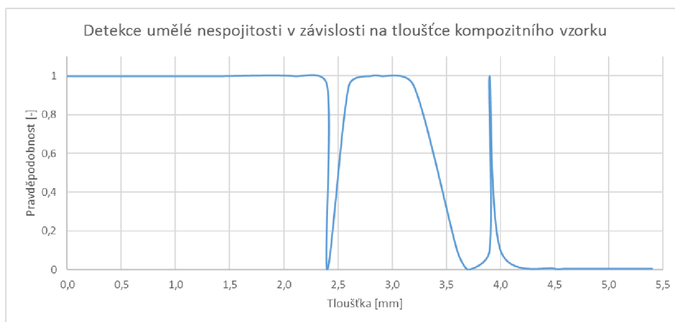
Graf 7.3 Křivka nalezení umělé nespojivosti sondy COMPROBE 10 MHz v závislosti na tloušťce materiálu
