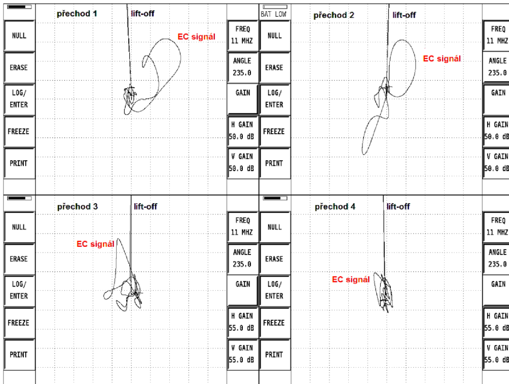
Obr. 7.16 Odezvy vířivých proudů jednotlivých přechodů pro pracovní frekvenci 11 MHz
