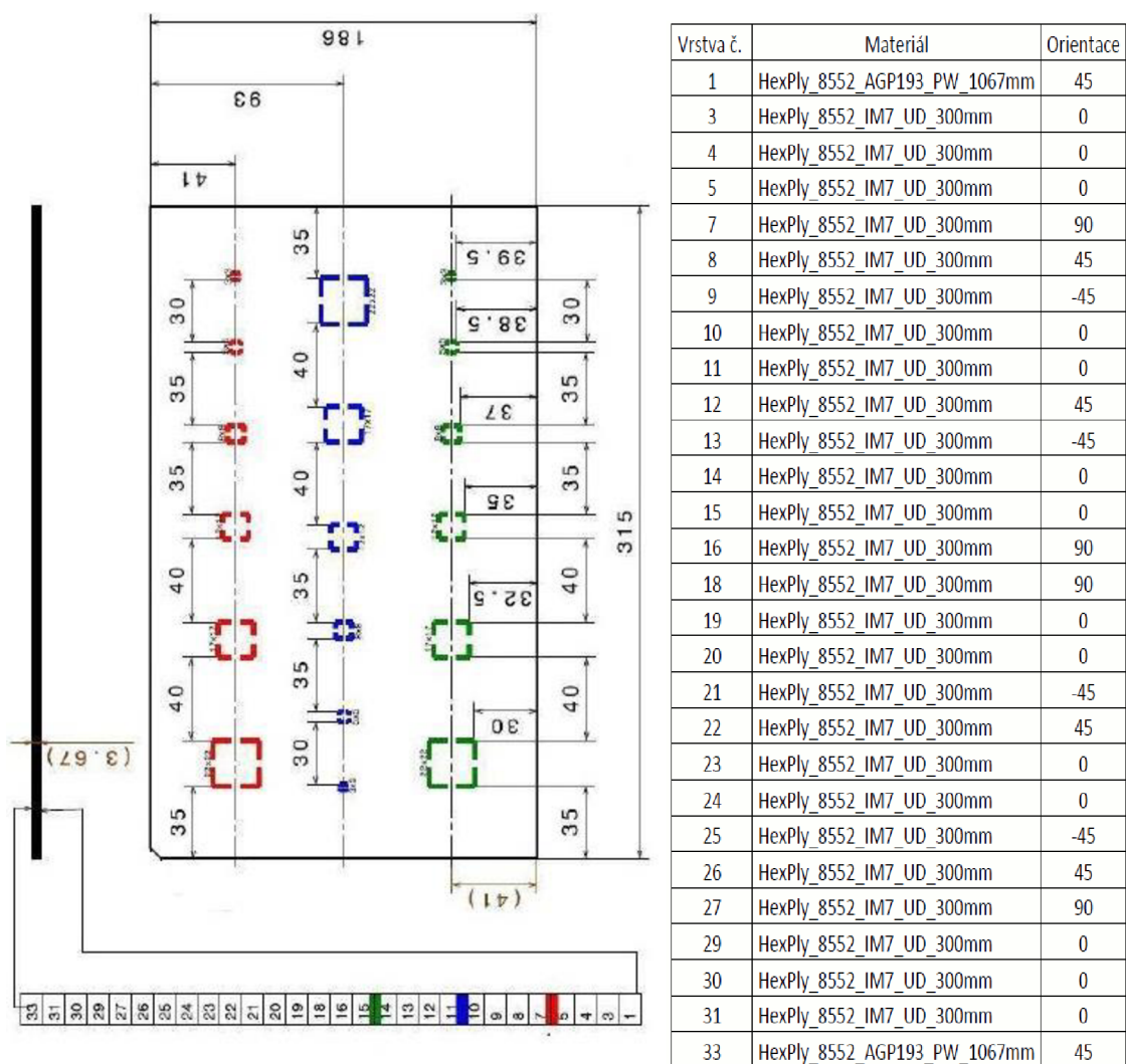
Obr. 6.6 Návrh vzorku 3 (vlevo), orientace a materiál jednotlivých kladených vrstev (vpravo) [16]
