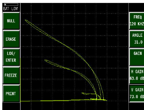
Obr. 3.4 Kalibrační vzorek pro povrchové zkoušení (vlevo), odezva vířivých proudů na vyjiskřené drážky (vpravo)
