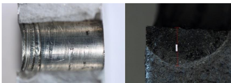
Obr. 3.10 Drážky po nástroji vzniklé při výrobě otvorů a vzniklá únavová trhlina
