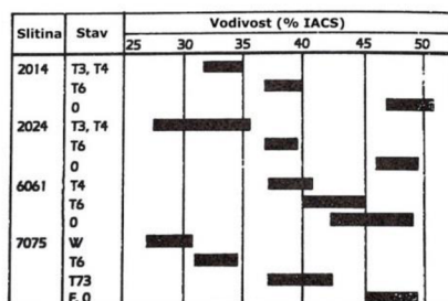
Obr. 3.18 Rozsahy vodivosti tvářených hliníkových slitin [7]
