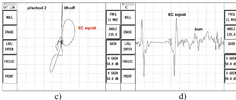
Obr. 7.17 Odezvy viřivých proudů v XY zobrazení pro přechod 2 pro: pracovní frekvence 7 MHz až 12 MHz (a), pracovní frekvenci 5 MHz (b), optimální pracovní frekvenci 11 MHz (c), EC signál v Yt zobrazení pro optimální pracovní frekvenci 11 MHz (d)
