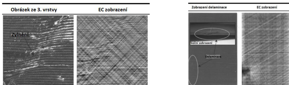
Obr. 3.26 Ukázka zvlnění ve 3. vrstvě (vlevo), delaminace (vpravo) [12]
