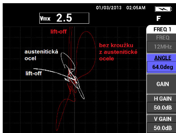
Obr. 7.34 EC signály jednotlivých stinících kroužků u sondy COMPROBE 10 MHz (přístroj Nortec 600D)
