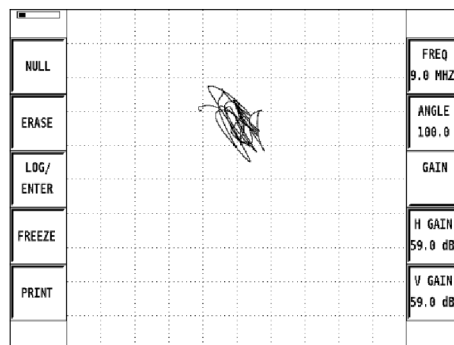
Obr. 7.6 EC signál uhlíkového prepegu bez defektu
