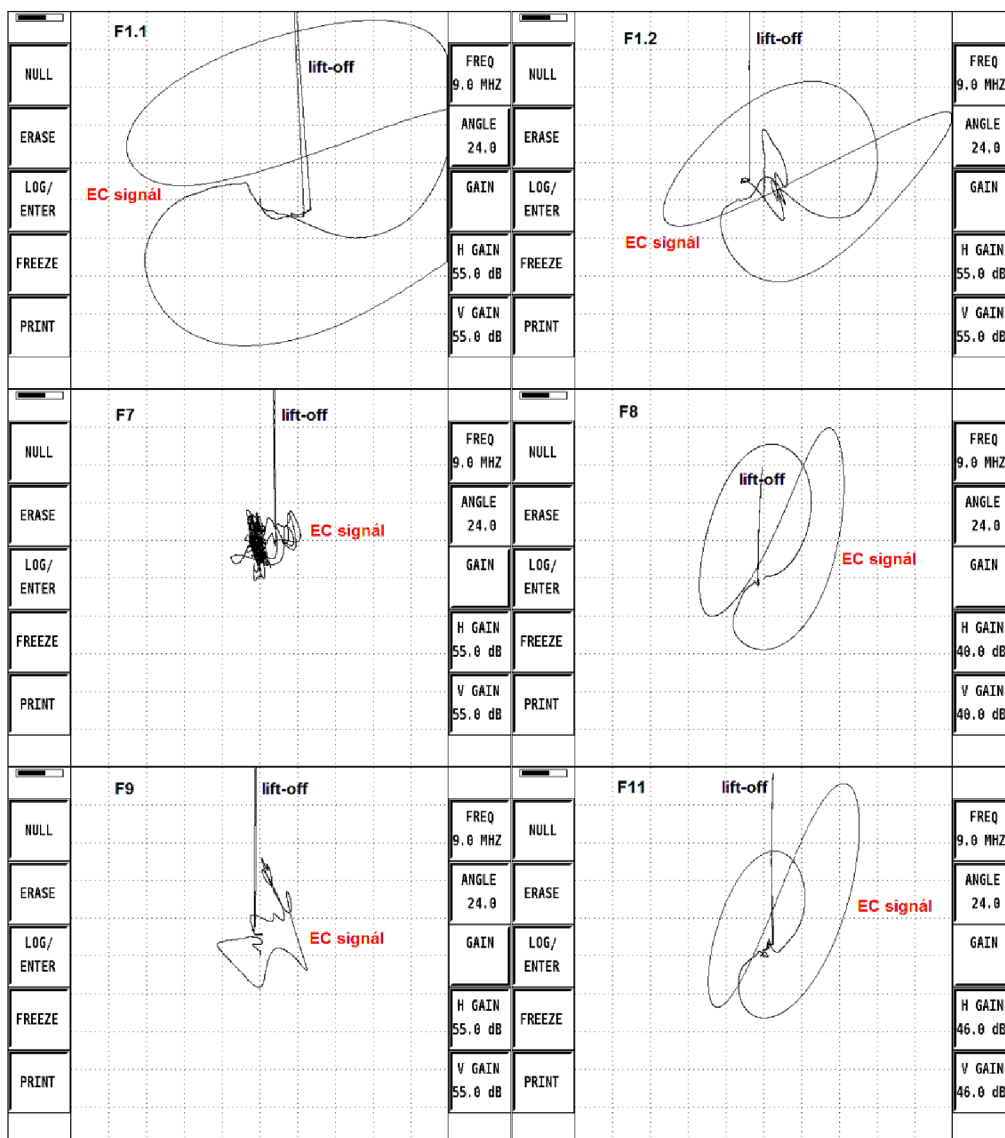
Obr. 7.20 EC signály jednotlivých detekovaných nespojitostí při pracovní frekvenci 9 MHz
