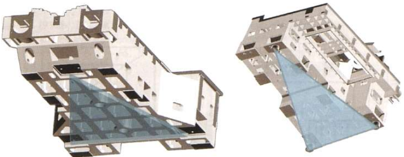
Obr. č. 27 Znárodnění tříbodového uložení samonosného rámu [1]
