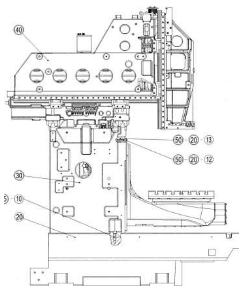
Obr. č. 41 Konstrukční provedení rámu frézky ecoMill50/DMU 50 [32]
