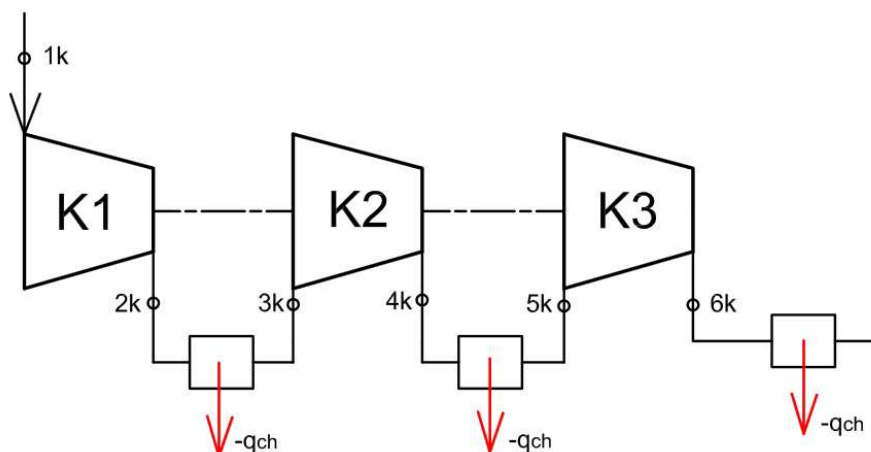
Obrázek 10.1 - Kompresní schéma
