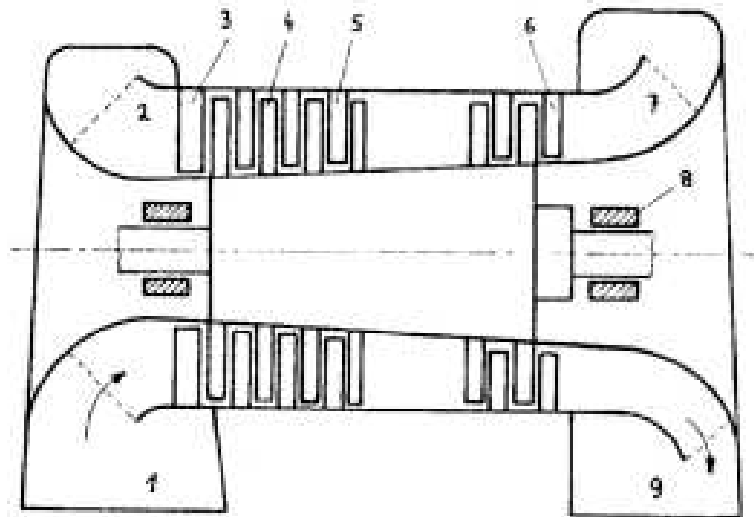
Obrázek 6.7 - Axiální kompresor [42]
