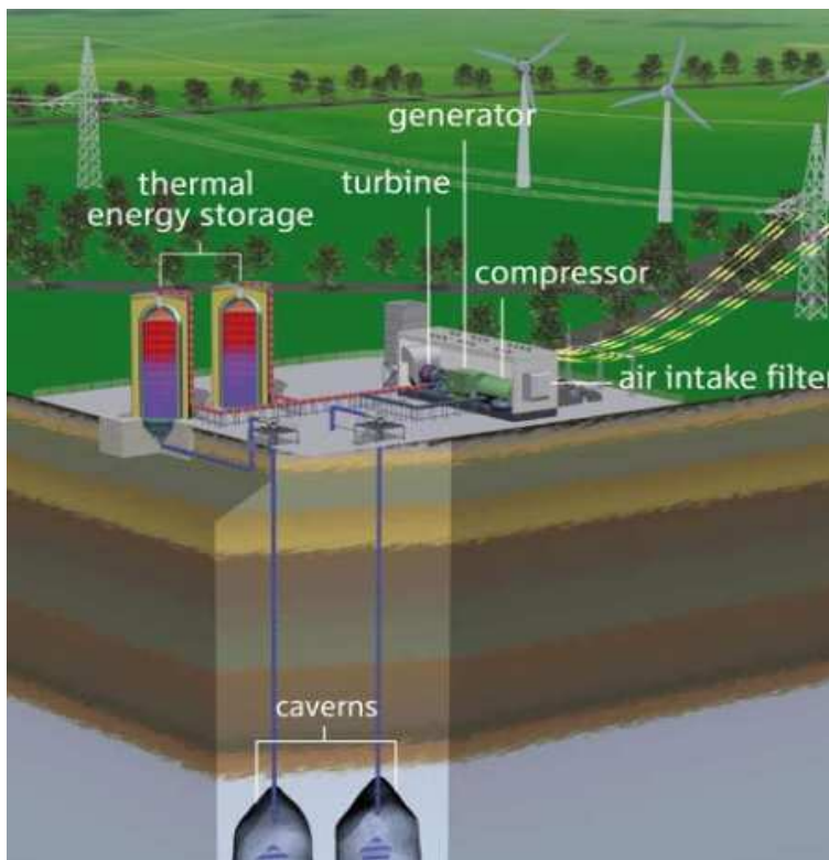
Obrázek 5.5 - Zařízení ADELE [9]
