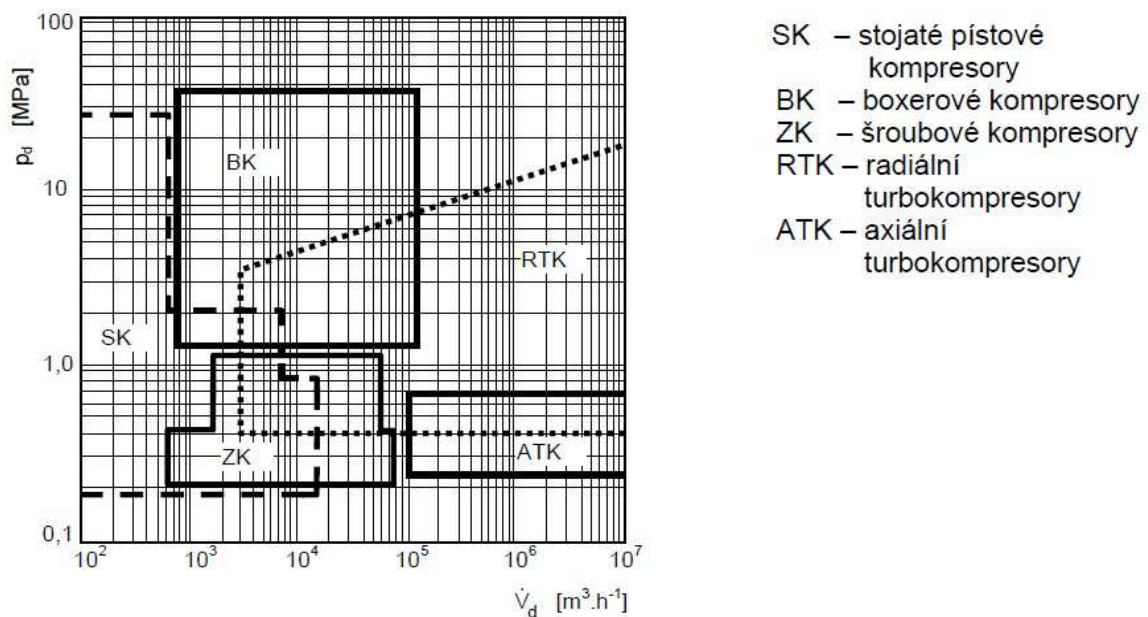
Obrázek 6.8 - Typy kompresorů podle parametrů [42]
