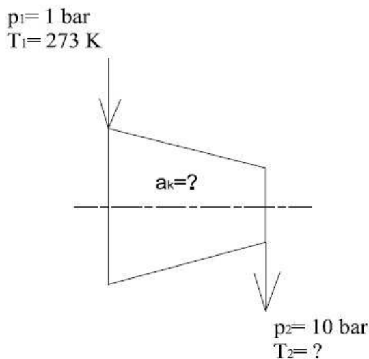
Obrázek 6.2 - Jednostupňová komprese
