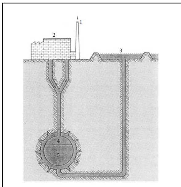
Obrázek 8.3 - Vyrovňovací zásobník [1]
