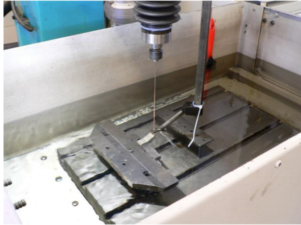
Obr. 15 – Elektroerozivní zařízení [51]
