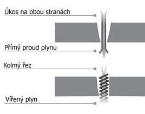
Obr. 23 – Vířivý a nevířivý paprsek [53]
