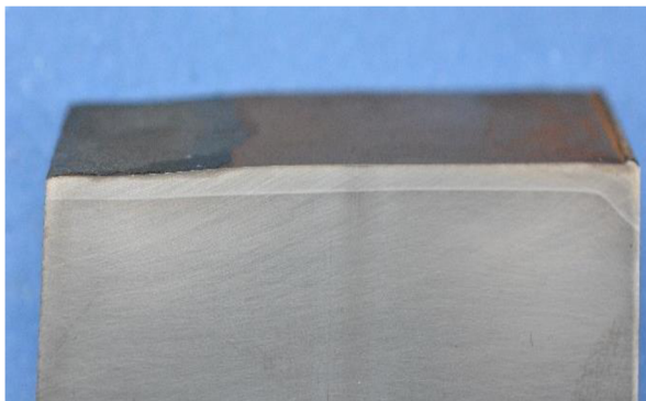
Obr. 52 – Šířka TOO tělesa T2-2: konec řezu. Naměřená šířka: 1,766 mm
