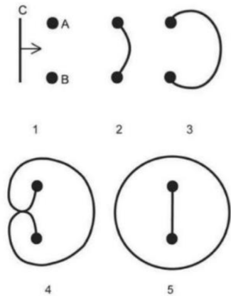
Obr. 7 – Frank-Readův zdroj dislokací [12]
