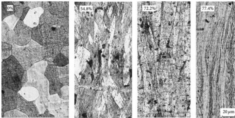
Obr. 6 – Přetvoření zastudena [10]
