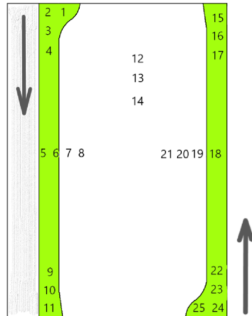
Obr. 38 – Poloha bodů pro měření tvrdosti povrchu tělesa T3 (XAR®). Řezná hrana T3-1 je na obrázku vlevo, řez T3-2 vpravo. Zelenou barvou jsou vyznačeny TOO řezů.
