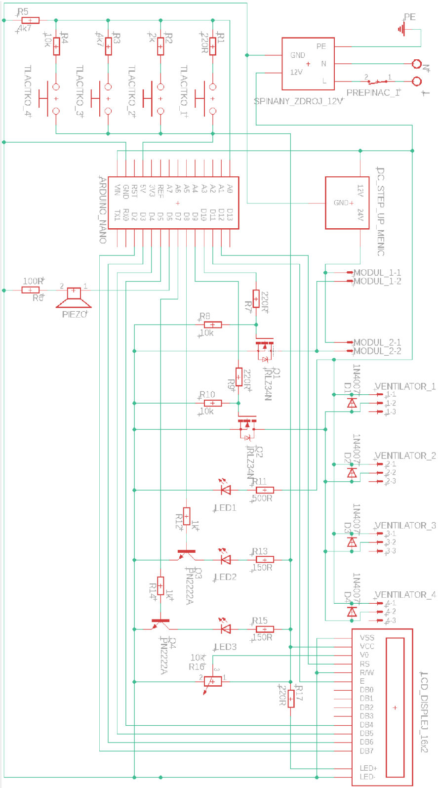
Priloha 1 - Schéma zapojení elektroniky
