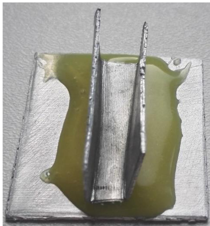
Obrázek 29 – Ukázka vzorku hliníku spojeného epoxidem
