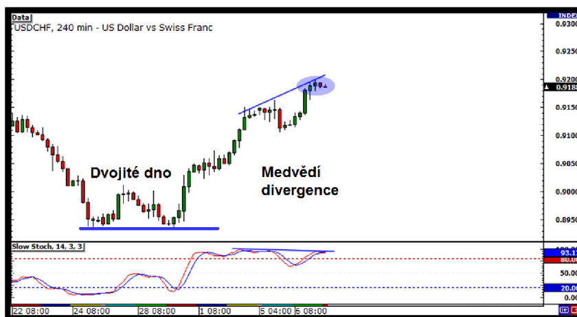
Obrázek 16: Medvědí divergenci
