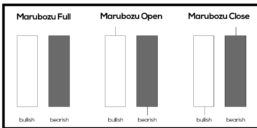
Obrázek 8: Marubozu
