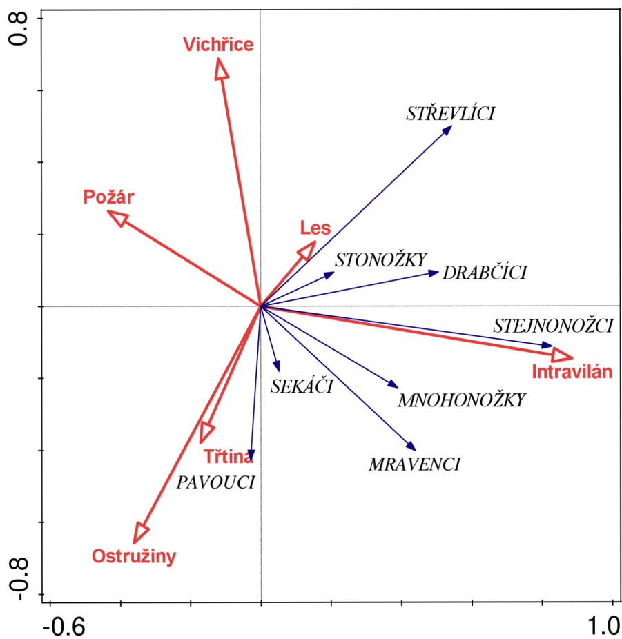
Obrázek 29 RDA biplot distribuce skupin sledovaných pomocí metody zemních pastí na Bradelské vrchovině. Environmentální faktory jsou zvýrazněné červeně.
