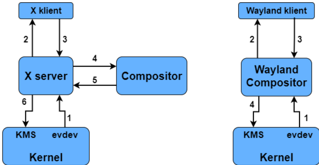
Obr. 1.1: Architektúra Wayland vs. X server[17]
