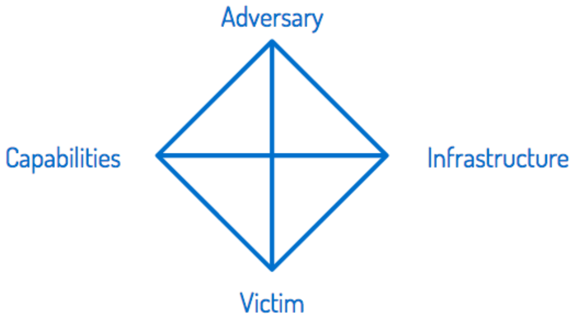
Obrázek 5: Diamond model [22]
