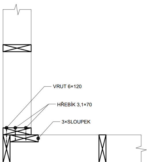
Obrázek 8 Rohový spoj č. 2
