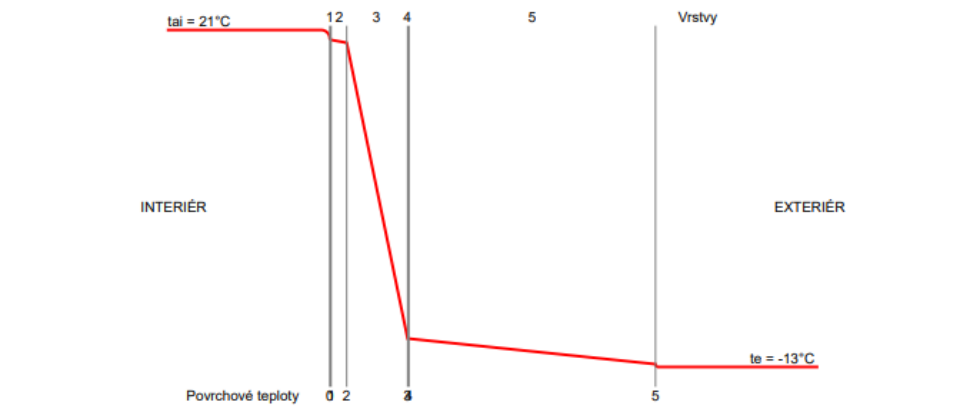
Graf 5 Průběh teplot v podlahové konstrukci [27]
