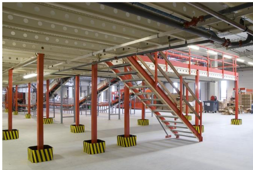
Obr. 1.4 Ukázka realizovaného vestavného podlaží
