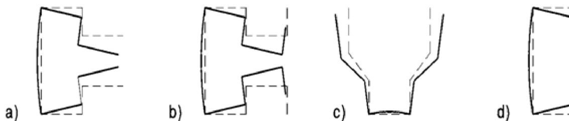
Obr. 2.13 Příklady distorzního vzpěru vybraných tvarů průřezu
