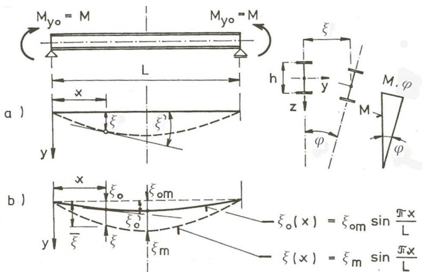
Obr. 2.7 Počáteční geometrické odchylky nosníku
