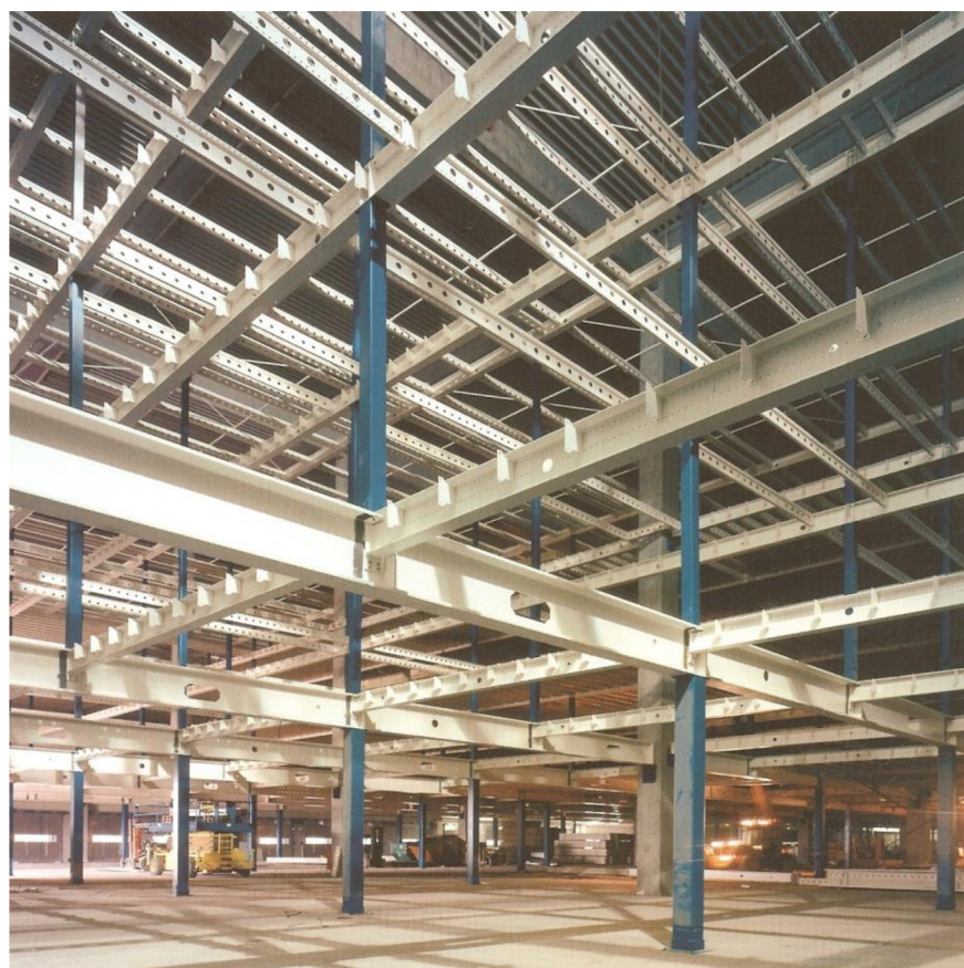
Obr. 1.5 Vestavné podlaží s primárními nosníky z hutních profilů
