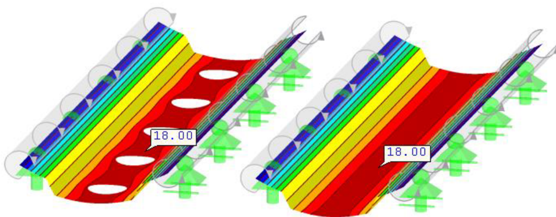
Obr. 5.6 Deformace modelů stojiny
