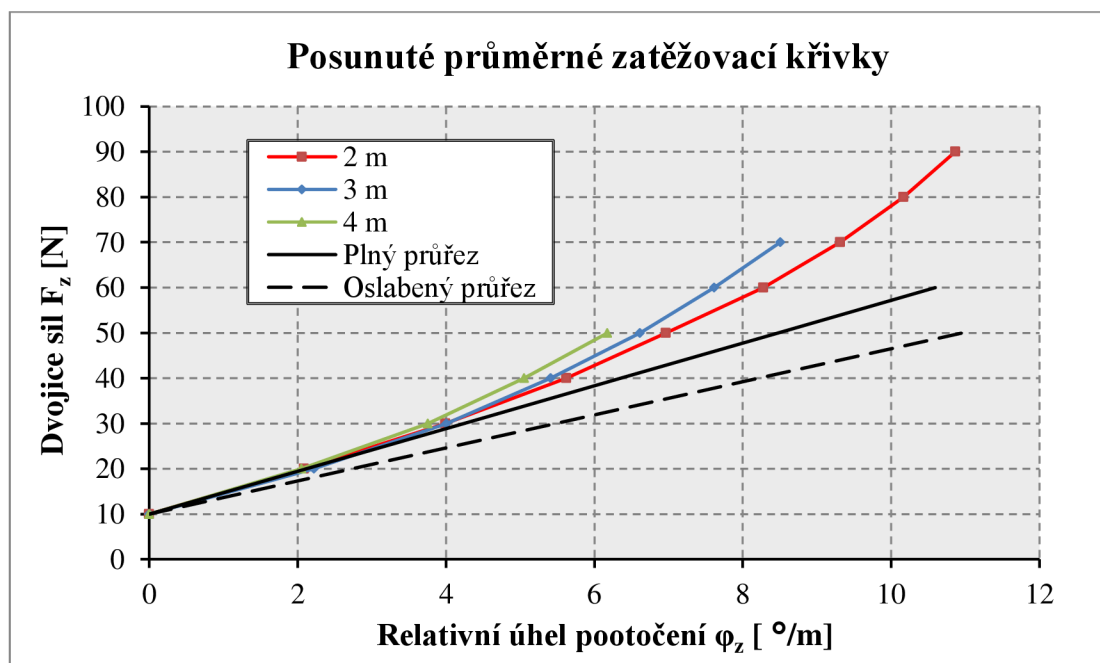
Graf 6.6 Posunutá průměrná zatěžovací křivky
