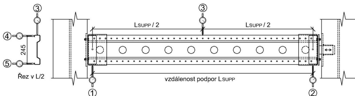
Obr. 6.36 Rozmístění snímačů deformací
