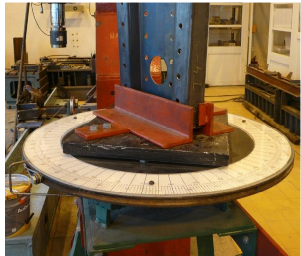
Obr. 6.10 Zatěžovací kotouč s unášecím pouzdem
