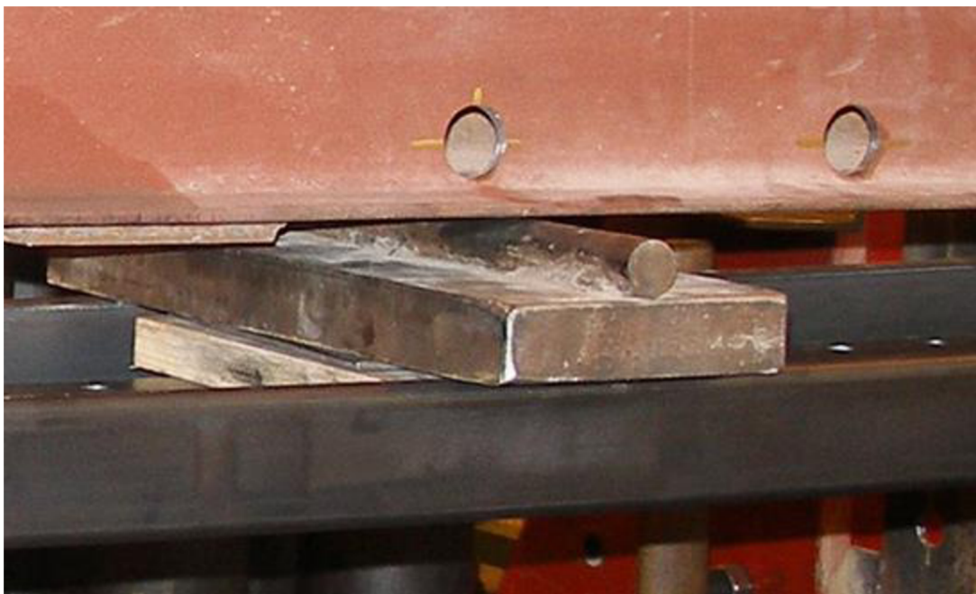
Obr. 6.23 Ocelová a dřevěná podložka – realizace
