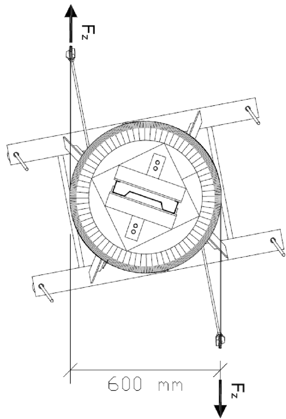
Obr. 6.7 Rameno dvojice sil F_z
