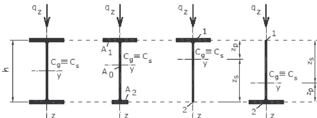
Obr. 2.2 Příklady průřezů 1. kategorie
