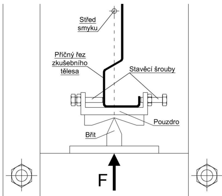
Obr. 6.35 Detail vnášení zatížení na spodní pásnici zkušební tělesa
