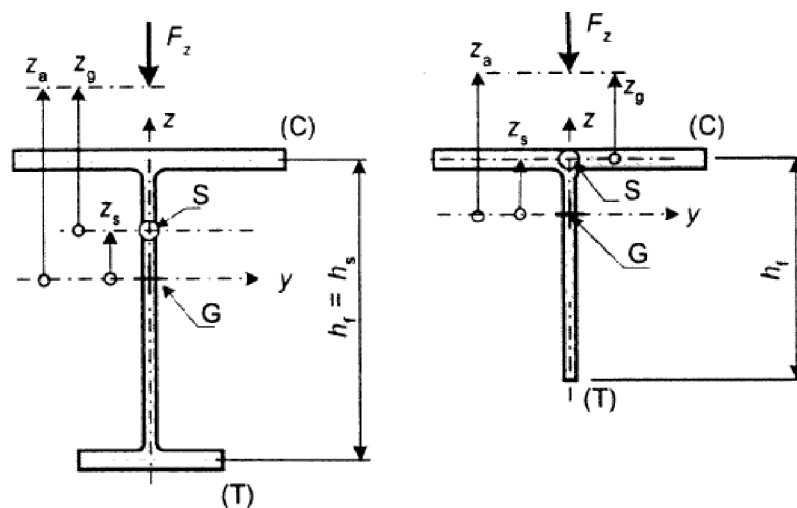
(C) tlačena vlákna, (T) tažena vlákna, S – střed smyku, G – těžiště
