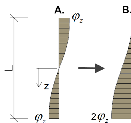
Obr. 6.15 Průběh zkroucení nosníku po jeho délce
