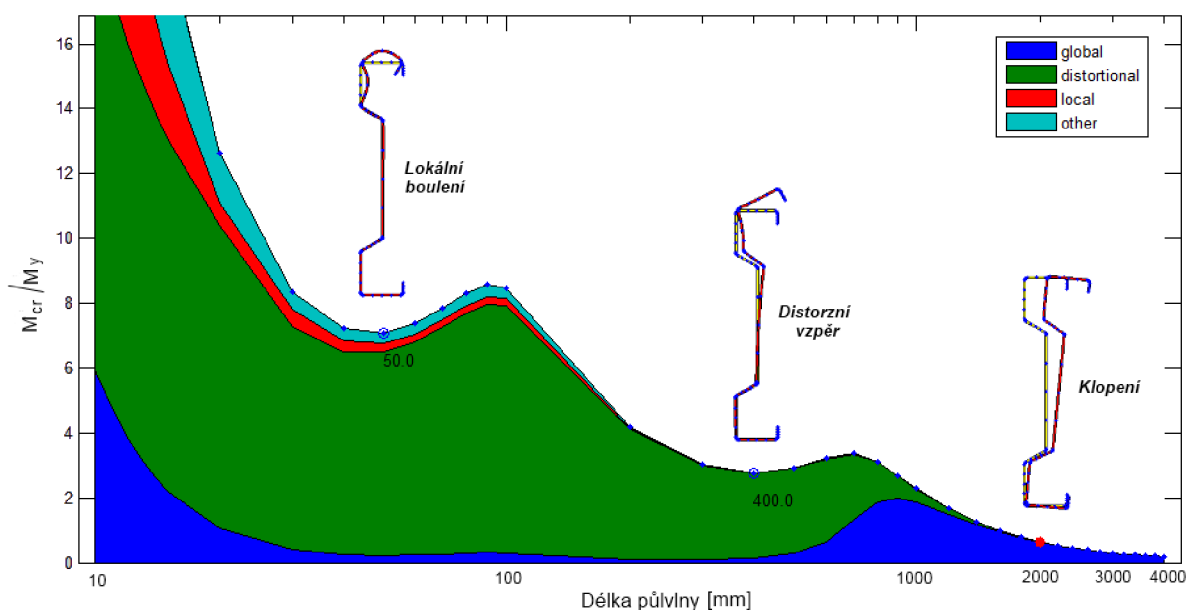
Obr. 5.3 Klasifikace jednotlivých stabilních jevů a jejich interakce
