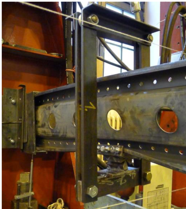
Obr. 6.41 Přičný ohyb pásnice v místě vnášení zatížení
