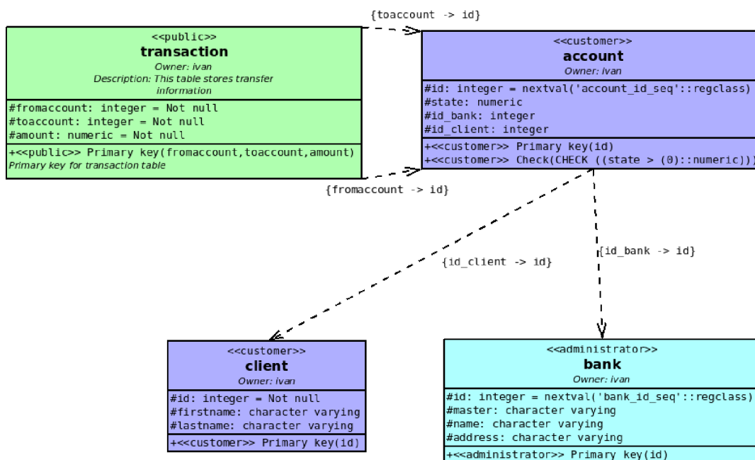
Obrázek 5.3: Výstupný diagram
