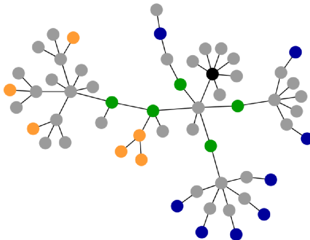
Obrázek 1.1: Príklad vizualizácie
