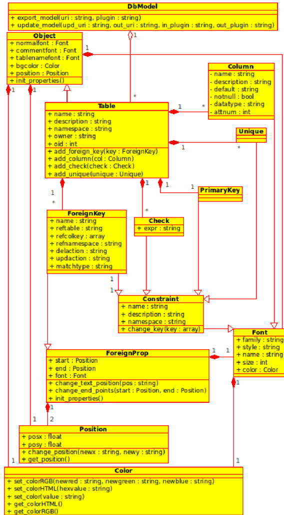
Obrázek 5.1: Diagram tried
