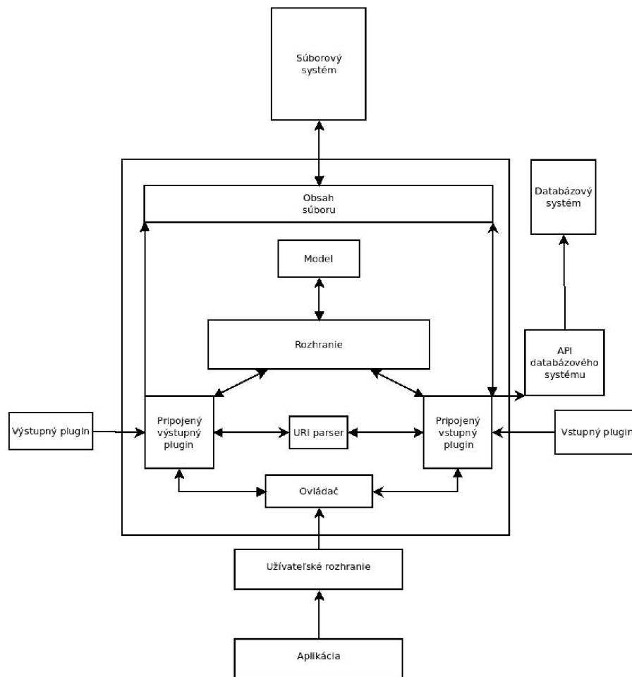
Obrázek 5.2: Architektúra knižnice
