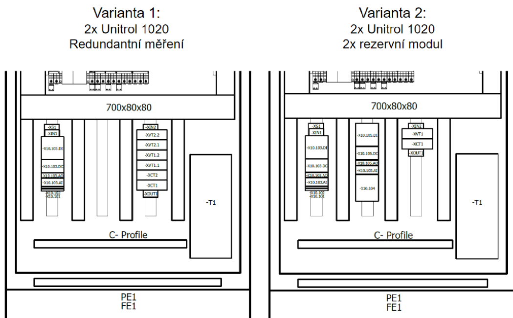
Obr. 6.9: Příklady variant v prostoru svorkovnic
