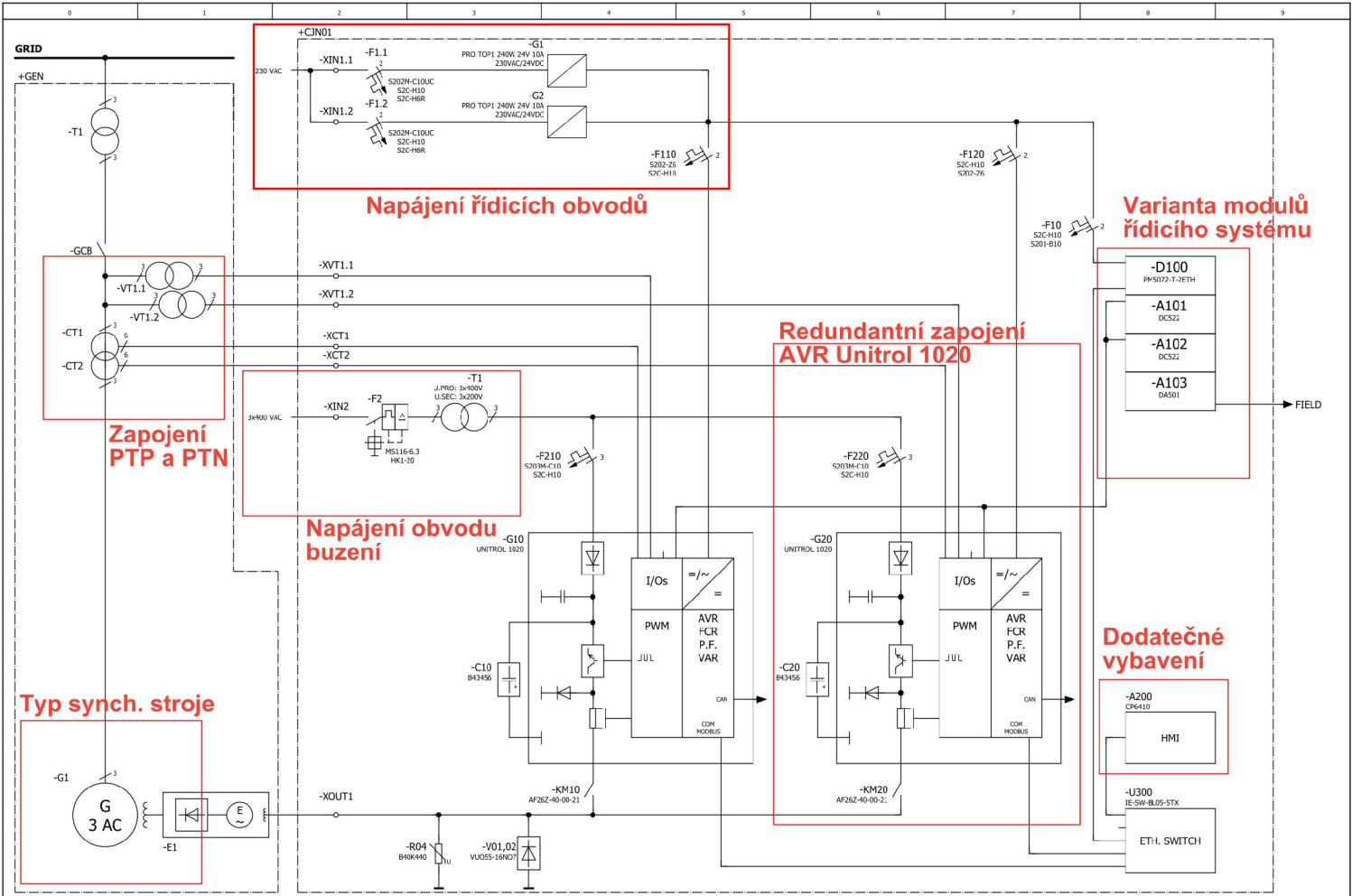
Obr. C.1: Popis oblastí blokového schéma
