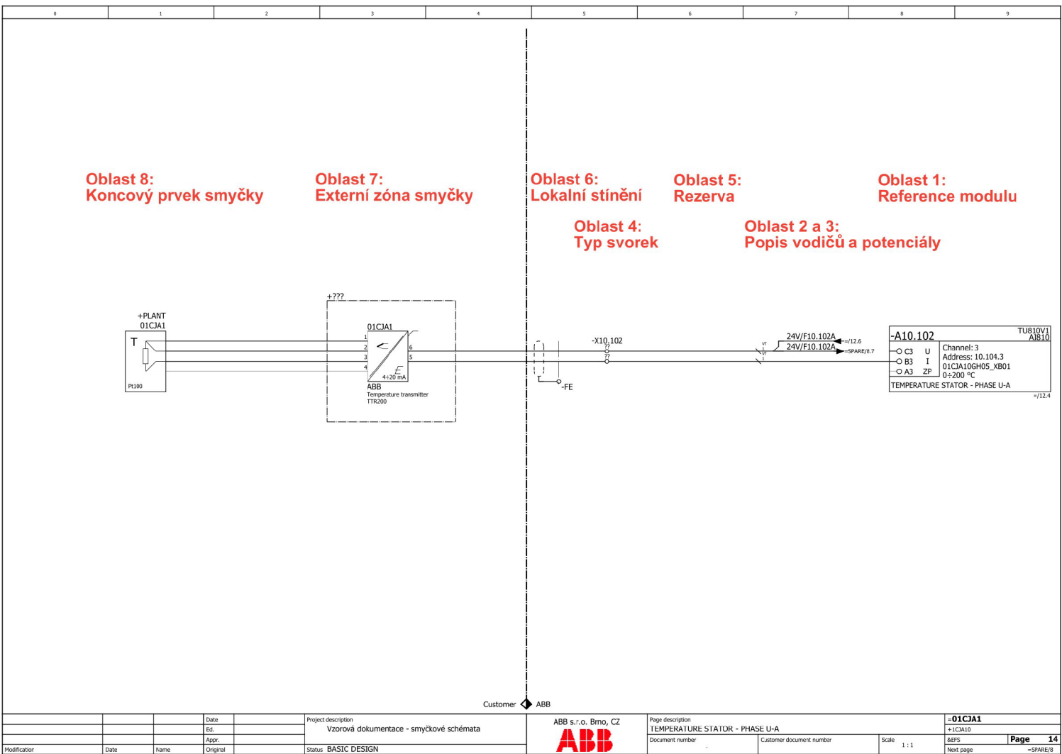
Obr. A.1.: Popis oblastí smyčkového schéma
