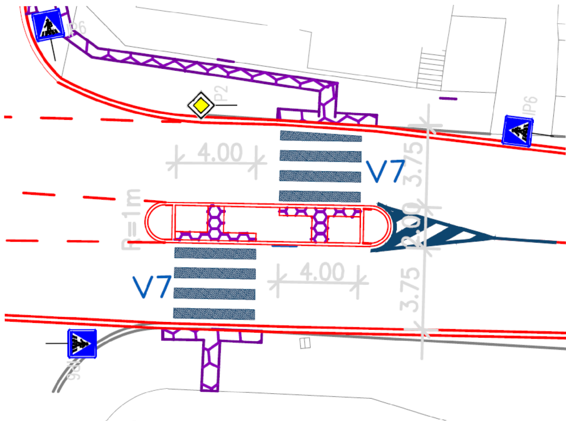
Obrázek 14: Návrh řešení v minulých letech – odsazený přechod pro chodce [6]
