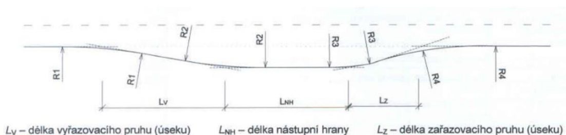
Obrázek 16: Normový obrázek – Navrhování zastávek [4]
