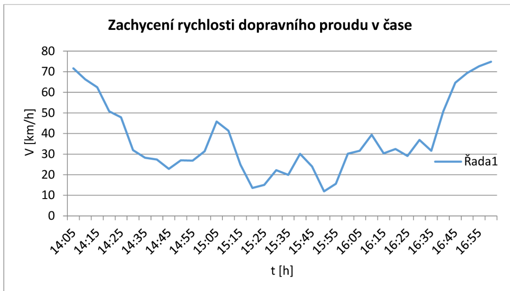
Obrázek 37: Zachycení rychlosti dopravního proudu v čase [31]
