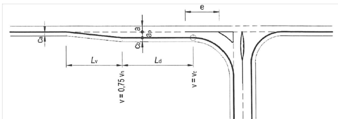
Obrázek 6: Přídavný pruh pro odbočení vpravo bez zastavení na úrovňové křižovatce[3]
