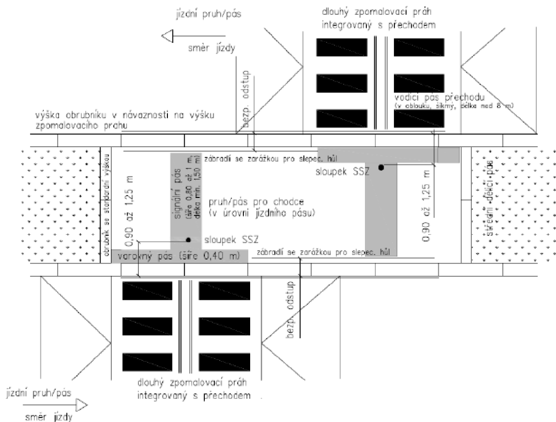
Obrázek 44: Odsazený přechod pro chodce [6]
