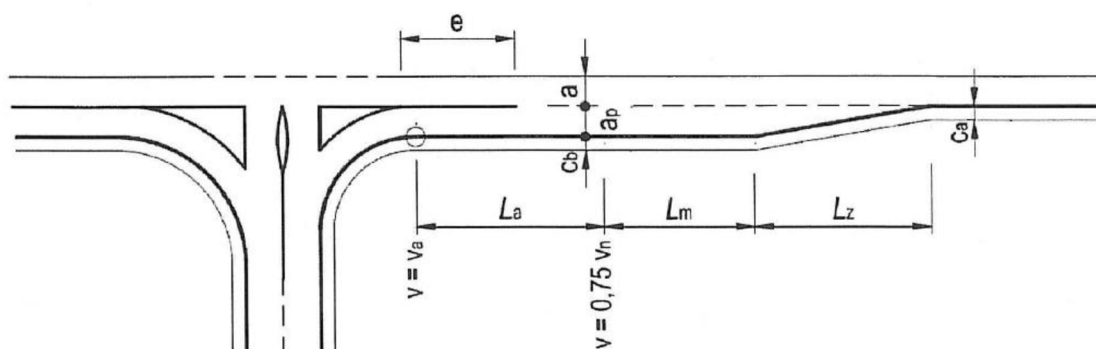
Obrázek 7: Příklad připojovacího pruhu na úrovňové křižovatce [3]
