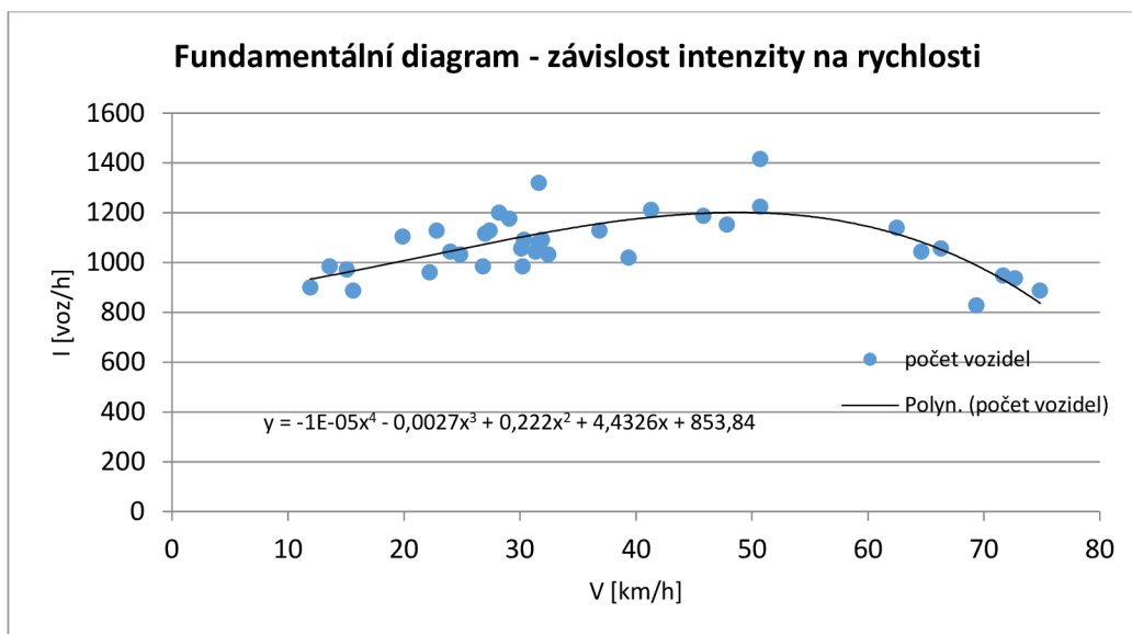
Obrázek 36: Fundamentální diagram (závislost intenzity na rychlosti) [31]
