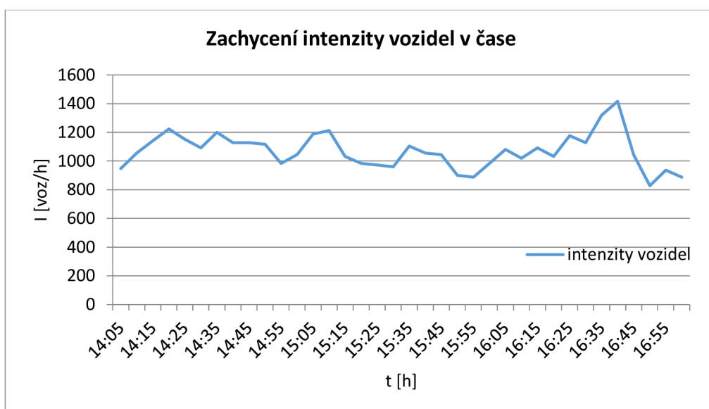
Obrázek 38: Zachycení intenzit vozidel v čase [31]
