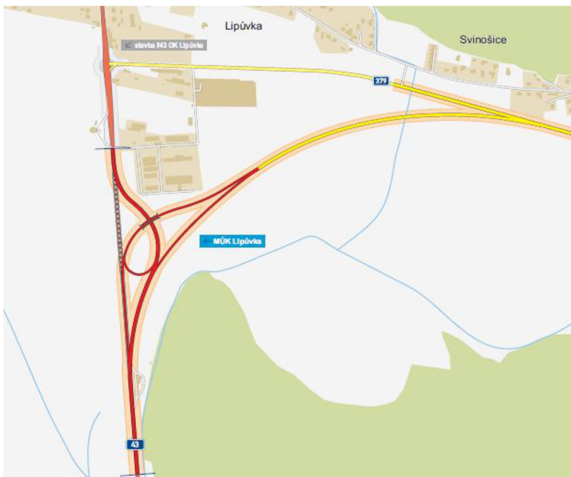
Obrázek 41: MÚK Lipůvka [35]
