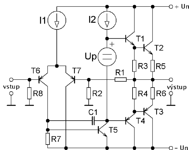
Obr. 1.10: Zjednodušené schéma výkonového zesilovače [2]
