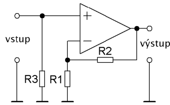
Obr. 1.1: Neinvertující zesilovač [8]
