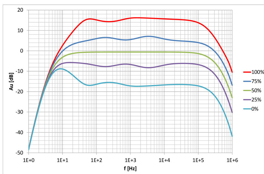
Obr. 4.1: Simulace f. char. vstupních jednotek č. 1 a 2
