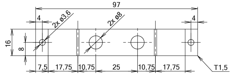
Výkres konstrukčních prvků pro mixážní pult David Krolák 2014 VUT BRNO
