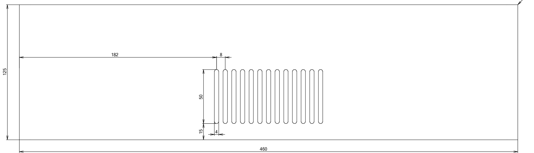
Výkres přední a zadní části přístrojové skříňky M1:2 David Krolák 2014 VUT Brno
