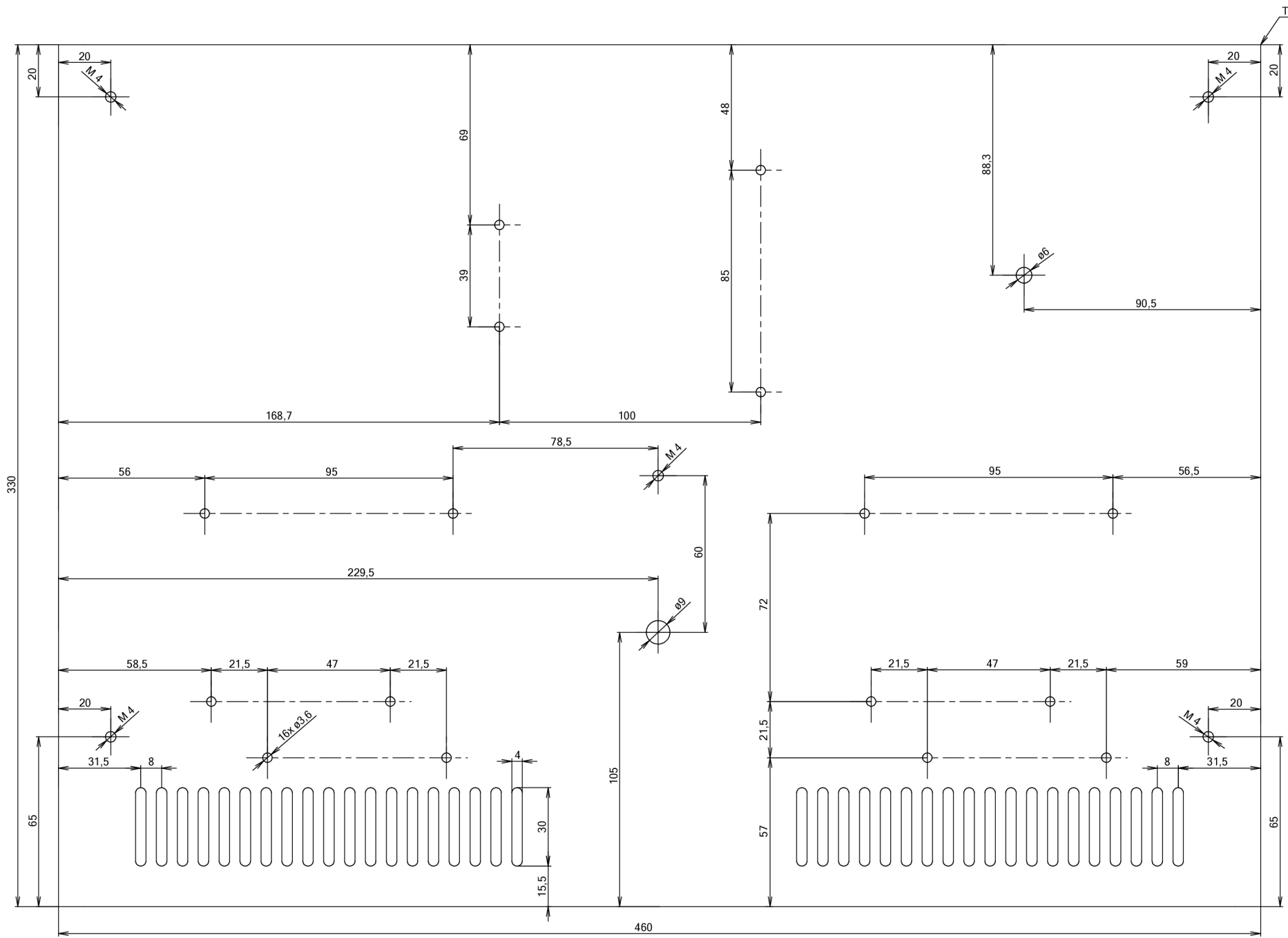
Výkres spodní části přístrojové skříňky M1:2 David Krolák 2014 VUT Brno
