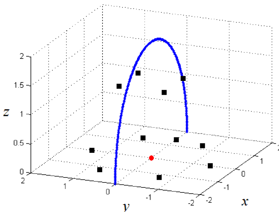
Obrázek 5.5: Trajektorie objektu zepředu dozadu (po oblouku) při konfiguraci 7.1.4
