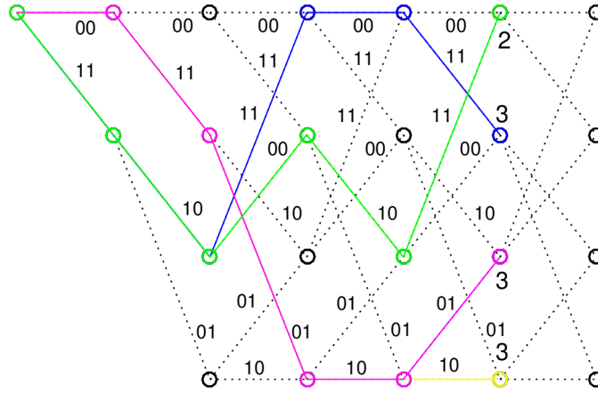
Obr. 1.16: Dekódování pomocí Viterbiho algoritmu 5. krok.
