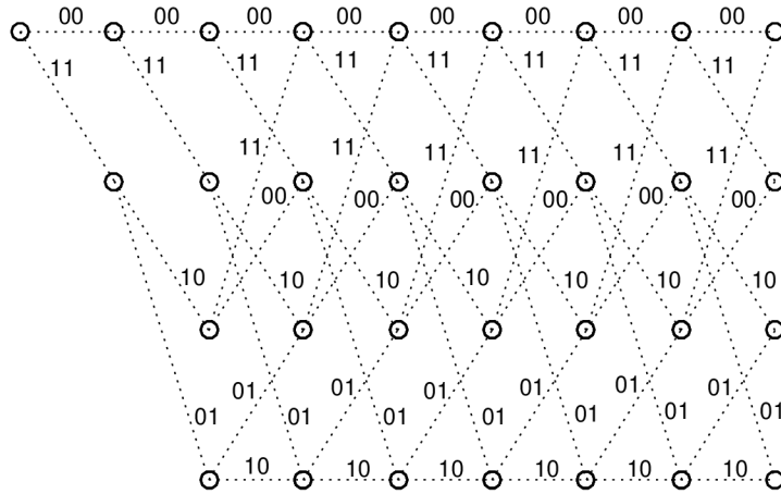
Obr. 1.10: Mřížový (trellis) diagram.
