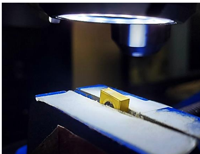
Obr. 26 Detail měření opotřebení destičky
