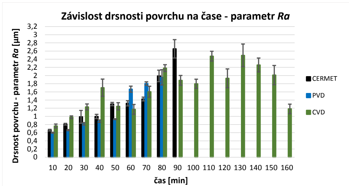
Obr. 42 Graf drsnosti povrchu - parametr R_a - při v_c = 200 \text{ m} \cdot \text{min}^{-1}
