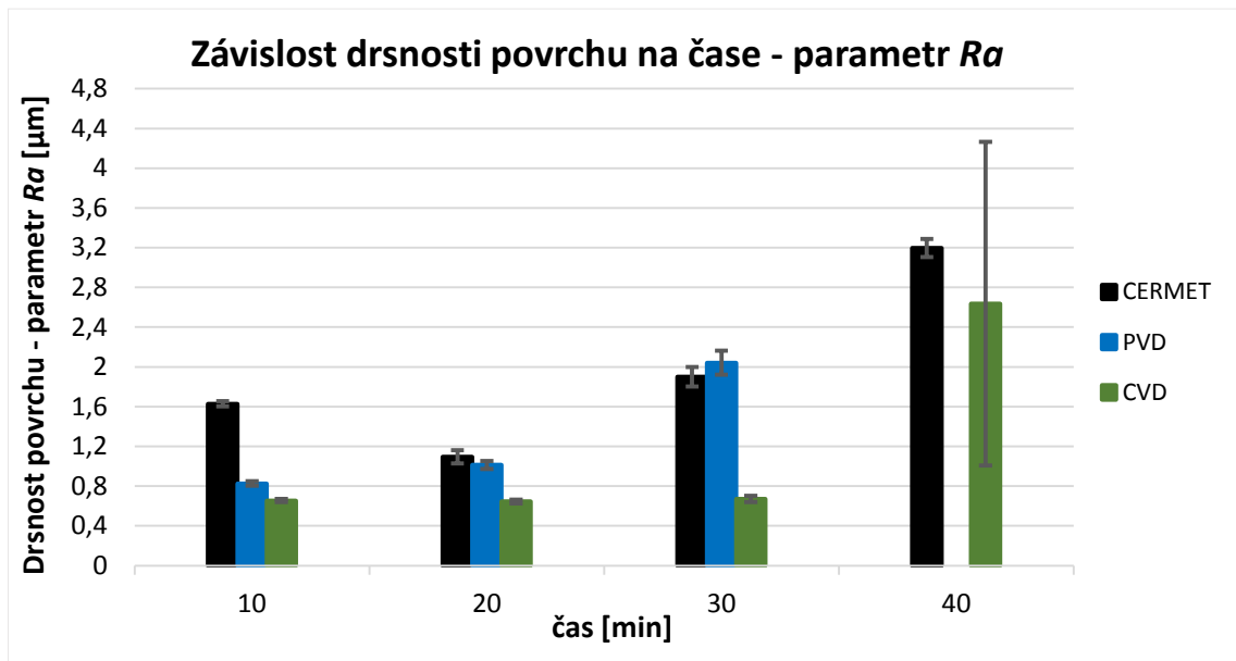
Obr. 44 Graf drsnosti povrchu - parametr Ra - při v_c = 300 \text{ m} \cdot \text{min}^{-1}
