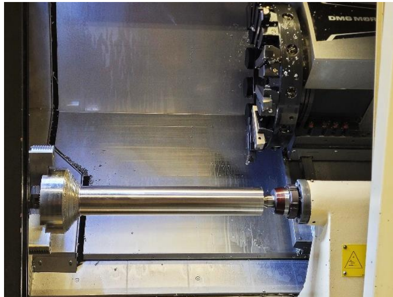
Obr. 20 Upnutí polotovaru
