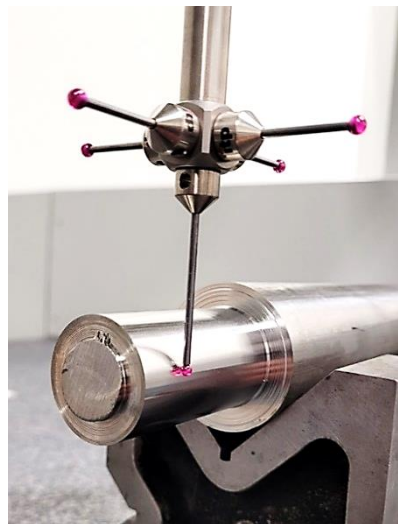
Obr. 29 Hvězdicový snímač
