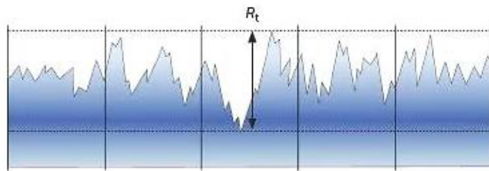
Obr. 13 Zobrazení vyhodnocování parametru R_t [19]
