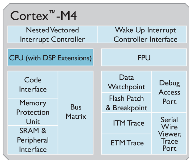
Obr. 4.4: Jádro ARM Cortex M4
