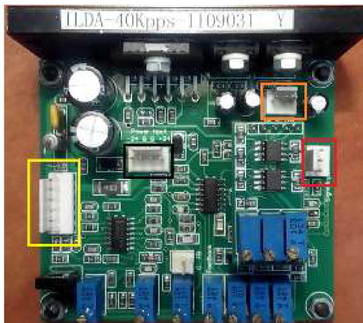
Obr. 6.5: Podpůrná deska k galvo motorům s vyznačenými piny pro připojení
