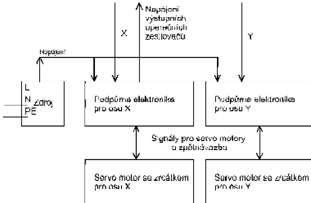
Obr. 6.4: Propojení galvo systému
