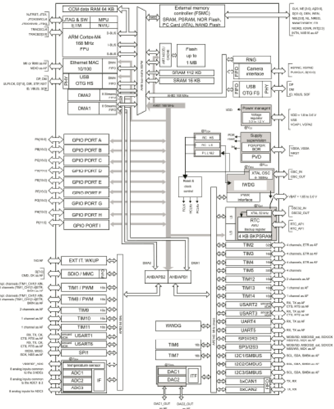
Obr. 4.3: Vnitřní zapojení STM32F407VGT6
