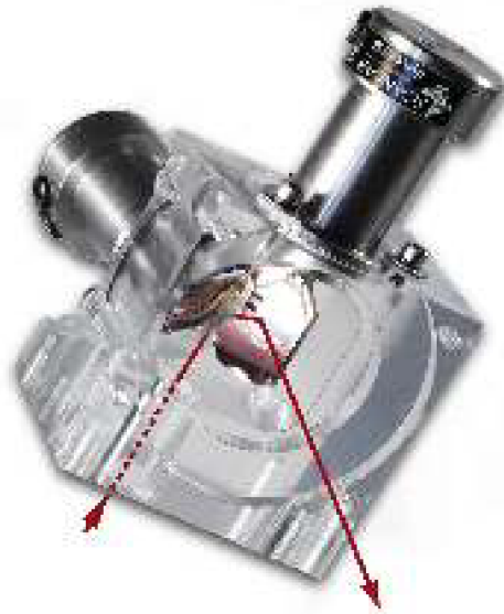
Obr. 4.2: Umístění galvo skenerů a průchod paprsku
