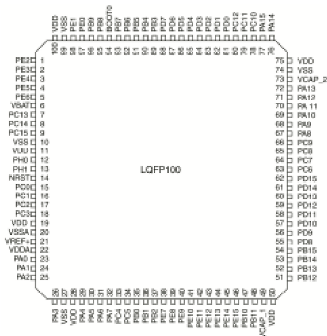
Obr. 3.3: Rozmístění pinů u vybraného STM32F407VGT6
