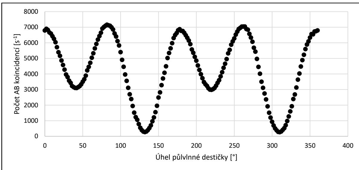
Obr. 4.4: Graf neupraveného čerpací svazku
