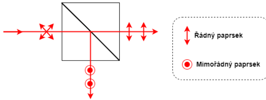
Obr. 1.1: Schéma funkce krychlového polarizačního děliče svazku (PBS) – svazek dopadající na PBS je lineárně polarizován s úhlem polarizace 45^\circ .
