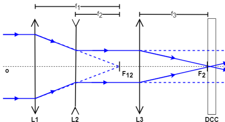
Obr. 3.8: Orientační schéma teleskopu vloženého do dráhy čerpacího paprsku pro zvýšení účinnosti konverze. Čočky L1 a L2 mají společné ohnisko F_{12} a zajišťují primární zúžení svazku, spojka L3 zaostruje paprsek na DC krystal; optická osa (o). Použité optické prvky: L1 (LA1229-B, f_1 = 175 mm), L2 (LC1715-B, f_2 = -50 mm), L3 (LA1464, f_3 = 1000 mm)
