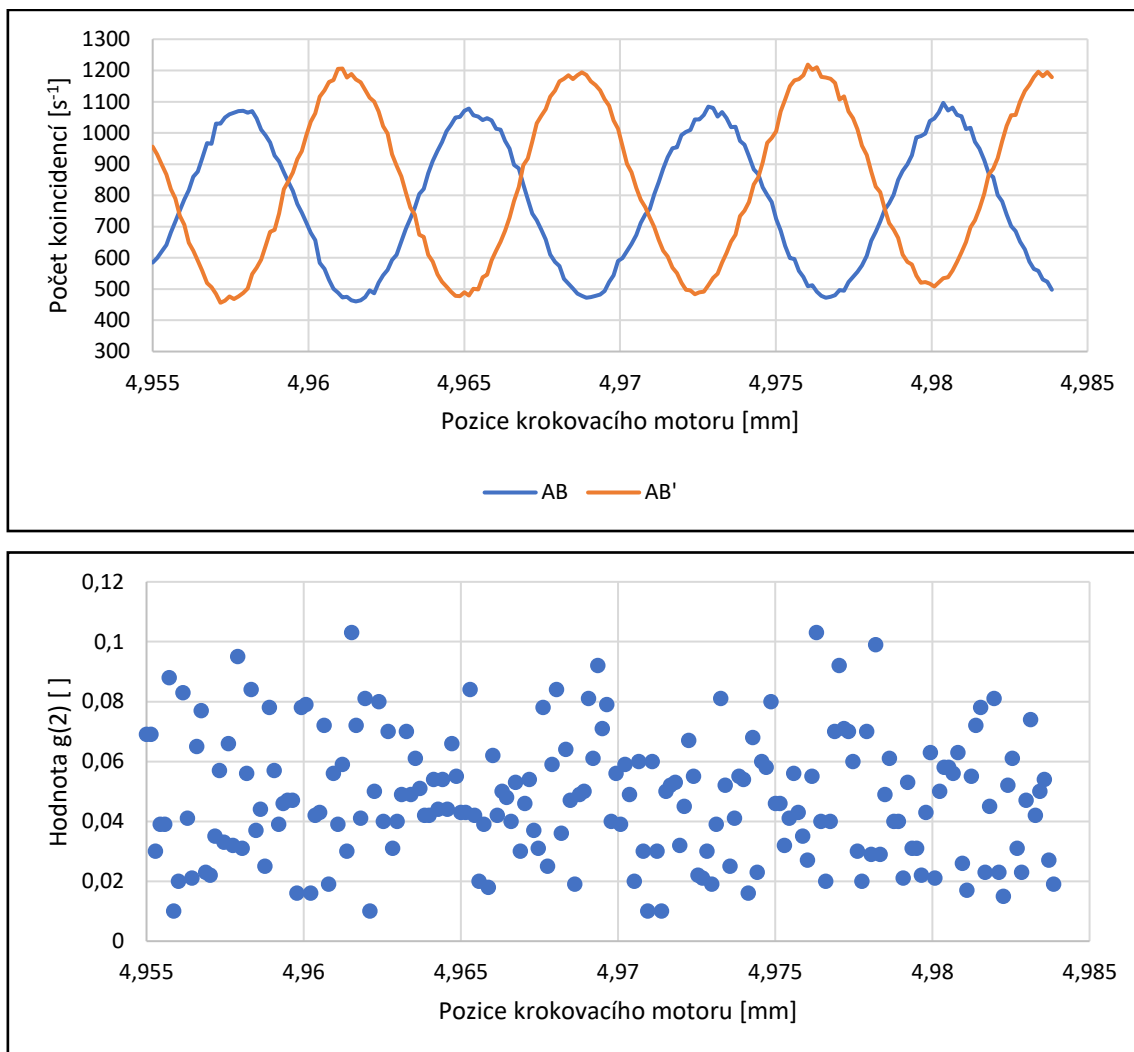
Obr. 4.19: Naměřený interferenční obrazec za počítání koincidence (nahore) a hodnota g^{(2)}(0) (dole) v rámci pokusu „Částice a vlny“
