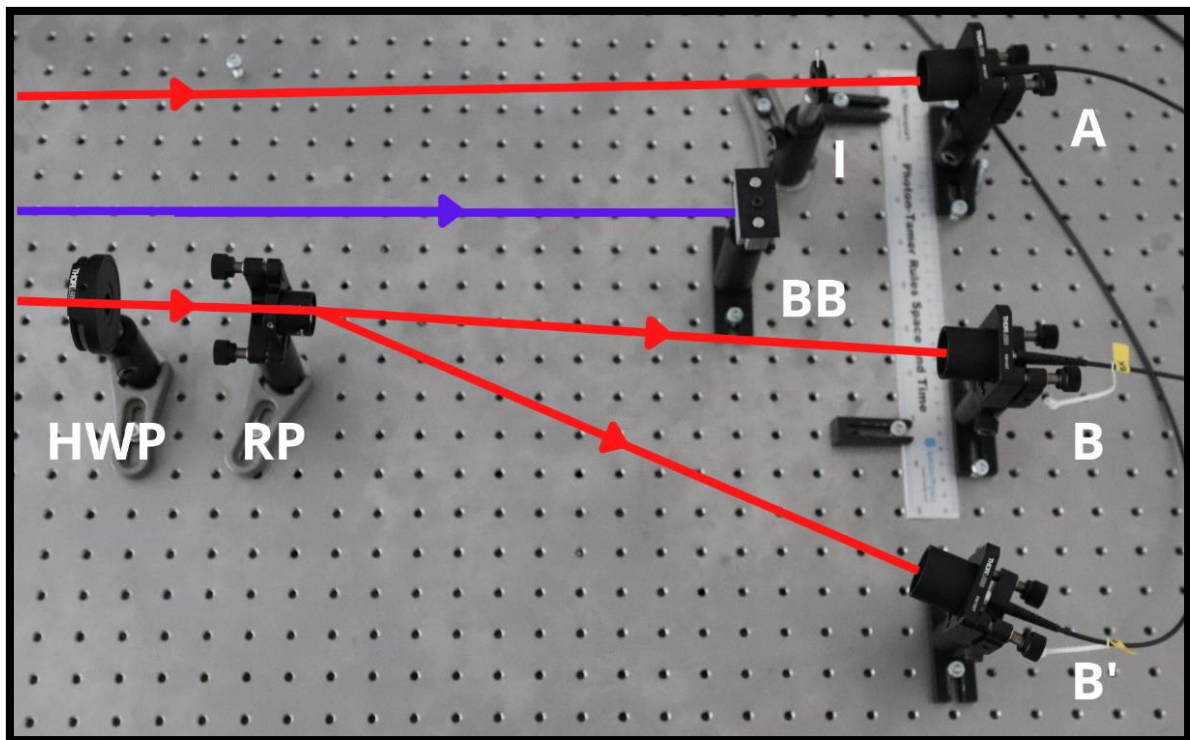
Obr. P2: Foto rozmístění optických prvků – Rochonův polarizátor. Na obrázku jsou paprsky (v příslušné barvě), sběrné optiky příslušných detektorů (A, B, B'), půlvlnná destička (HWP), Rochonův polarizátor (RP), clonka (I), pohlcovač svazku (BB).
