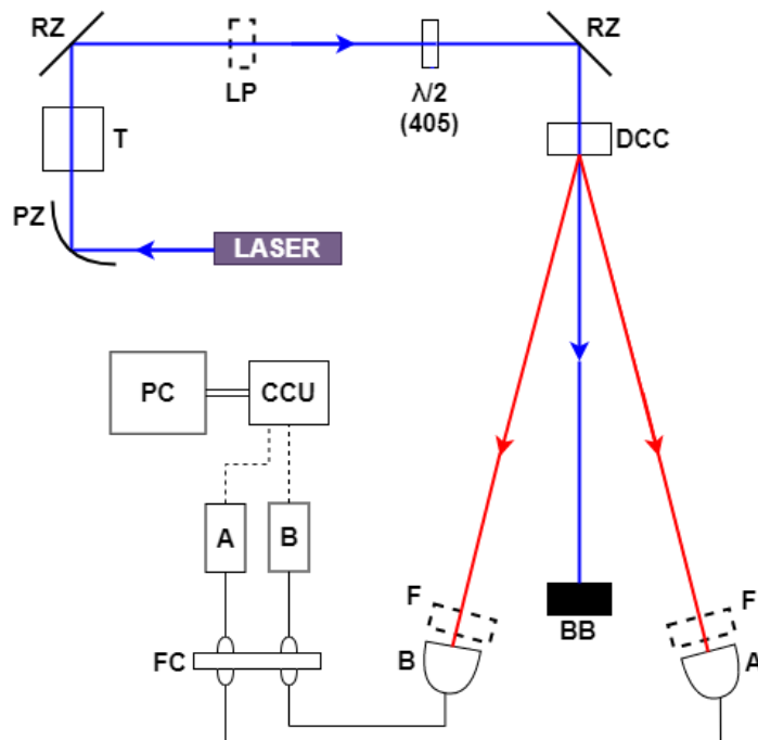
Obr. 3.1: Schéma sestavy pro SPDC. Schéma zachycuje základní optické prvky, tedy zdroj čerpacího paprsku (LASER), parabolické zrcadlo (PZ), teleskop upravující průřez svazku (T), rovinná zrcadla (RZ), lineární polarizátor (LP), půlvlnná destička s příslušnou vlnovou délkou ( \lambda/2 ), sestupně konverzní krystal (DCC), pohlcovač svazku (BB), umístění úzkopásmových filtrů (F) sběrnou optikou vedoucí na příslušný detektor (A, B), spojení optických kabelů (FC), koincidenční jednotka (CCU) a osobní počítač (PC).
