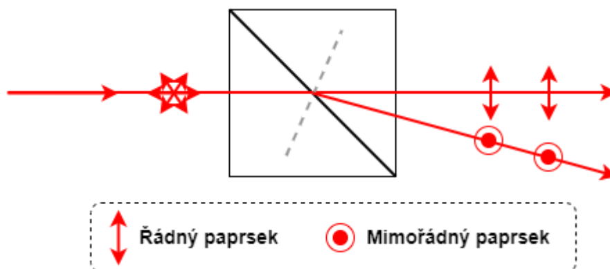
Obr. 2.4: Schéma Rochonova polarizátoru, vlastní tvorba podle [21]
