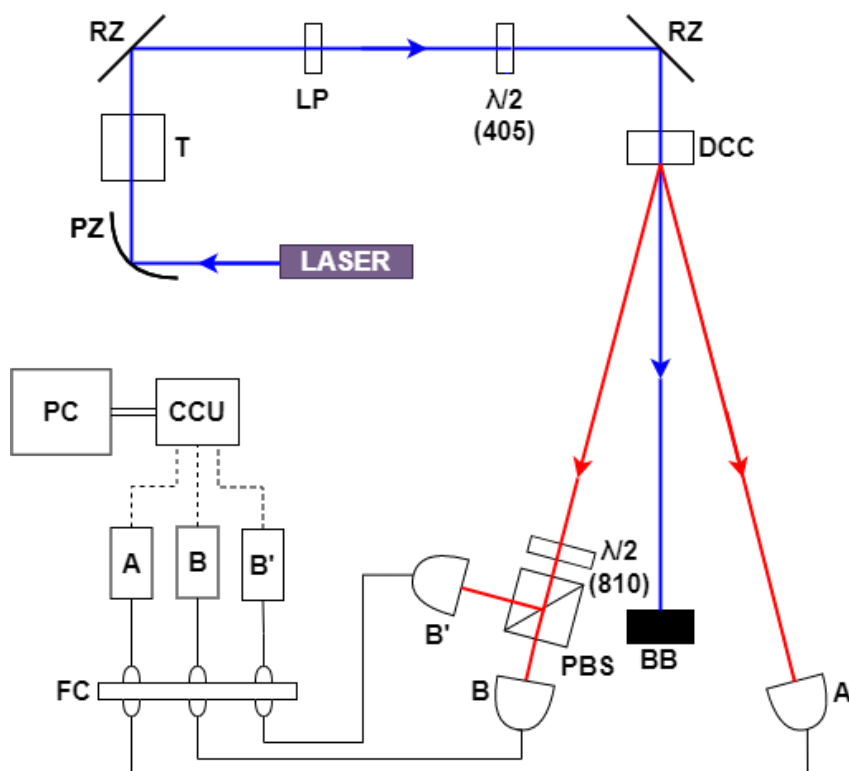
Obr. 3.2: Schéma sestavení experimentu Důkaz existence fotonů . Schéma odpovídá obr. 3.1,
