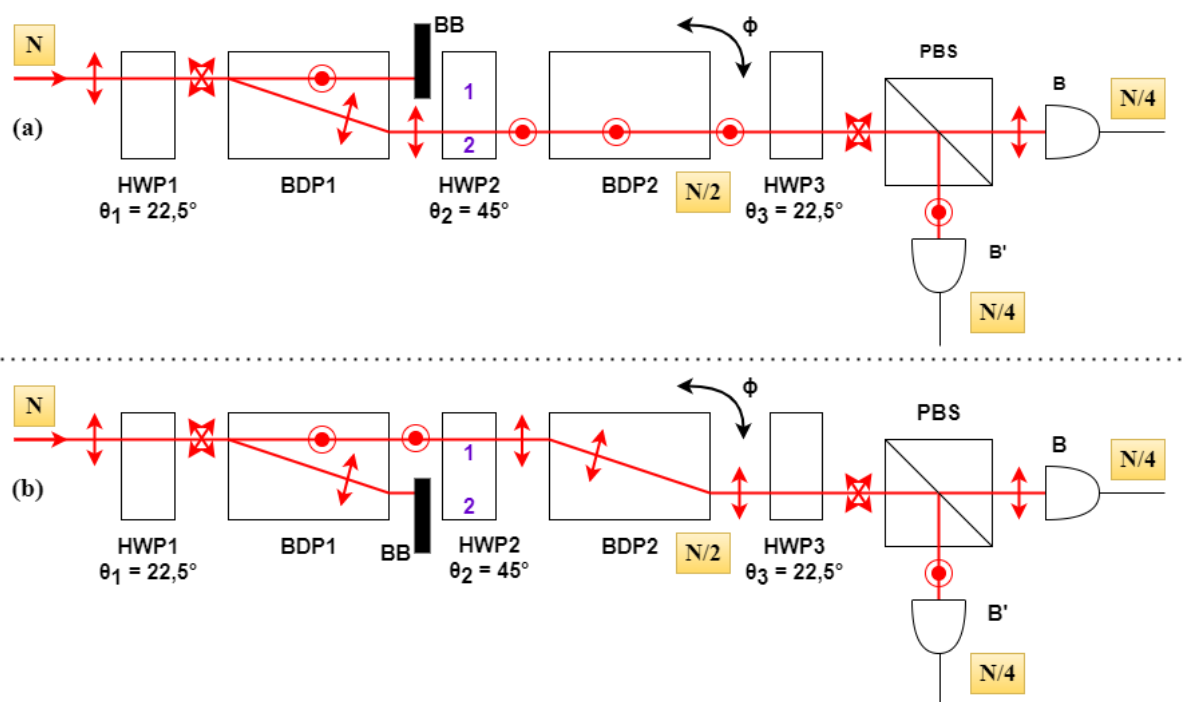
Obr. 3.6: Varianty experimentu s blokáci cest interferometrem, kdy nedochází k interferenci: (a) blokáce cesty 1, (b) blokáce cesty 2. Popis odpovídá obr. 3.5, černě je zaznamenáno zaslepení svazku (překážka), množství detekovaných fotonů na detektorech B a B' odpovídá čtvrtině vstupního množství.
