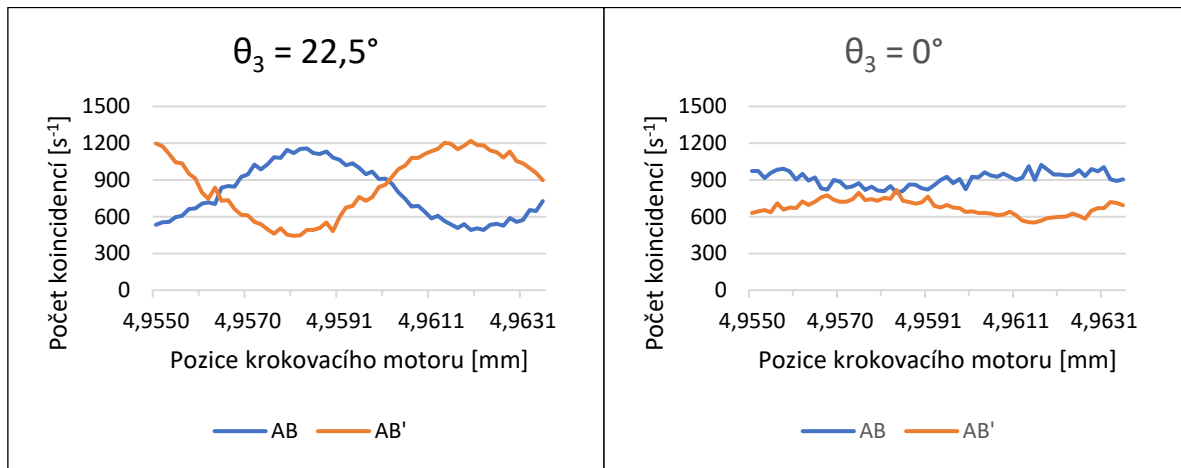
Obr. 4.17: Proměření jedné periody interference při změně natočení půlvlnné destičky (HWP3) \theta_3 = 22,5^\circ (vlevo), \theta_3 = 0^\circ (vpravo)
