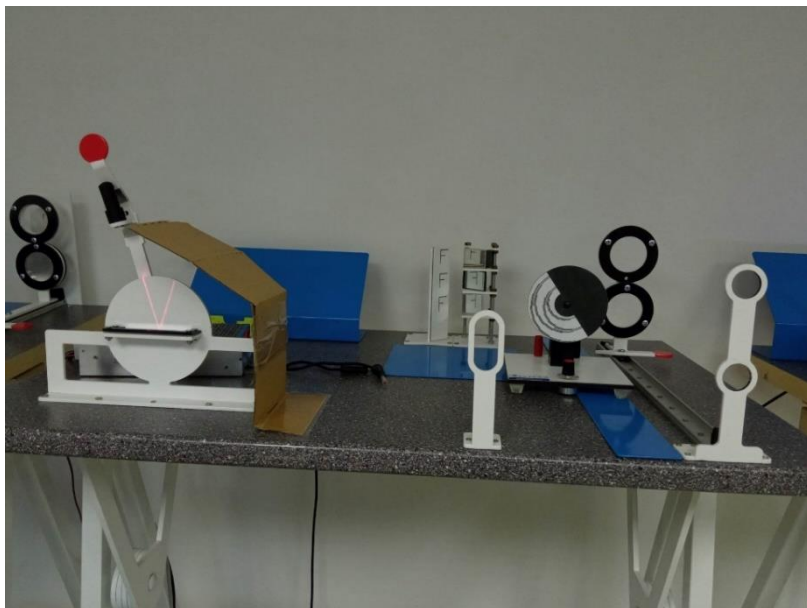
Obr. č. 17: Optická lavice – zrcadla. Foto autor
