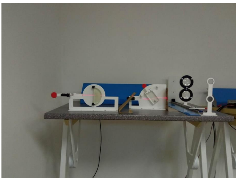
Obr. č. 18: Optické lavice – lom světla. Foto autor
