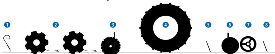
Obrázek 4: Schéma částí secího stroje Falcon 8 PRO Ferth+ QH (Farmet a.s.).
