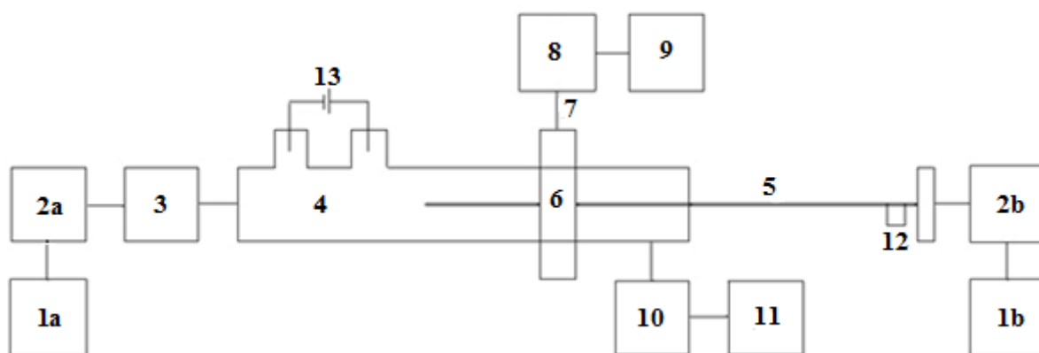
Obrázek 4: Schéma aparatury: 1a – tlaková láhev s kapalným dusíkem 6.0, 1b – tlaková láhev s kapalným dusíkem 5.0, 2a – regulátor hmotnostního průtoku (průtok 2000 ml/min), 2b – regulátor hmotnostního průtoku (průtok 7,5 ml/min), 3 – katalyzátor Oxiclear, 4 – výbojová trubice z křemenného skla QUARTZ, 5 – trubice ze skla PYREX, 6 – posuvný jezdec, 7 – optický kabel, 8 – spektrometr, 9 – PC, 10 – vymrazovací nádoba s kapalným dusíkem, 11 – rotační olejová vývěva, 12 – nádoba se vzorkem, 13 – zdroj napětí
