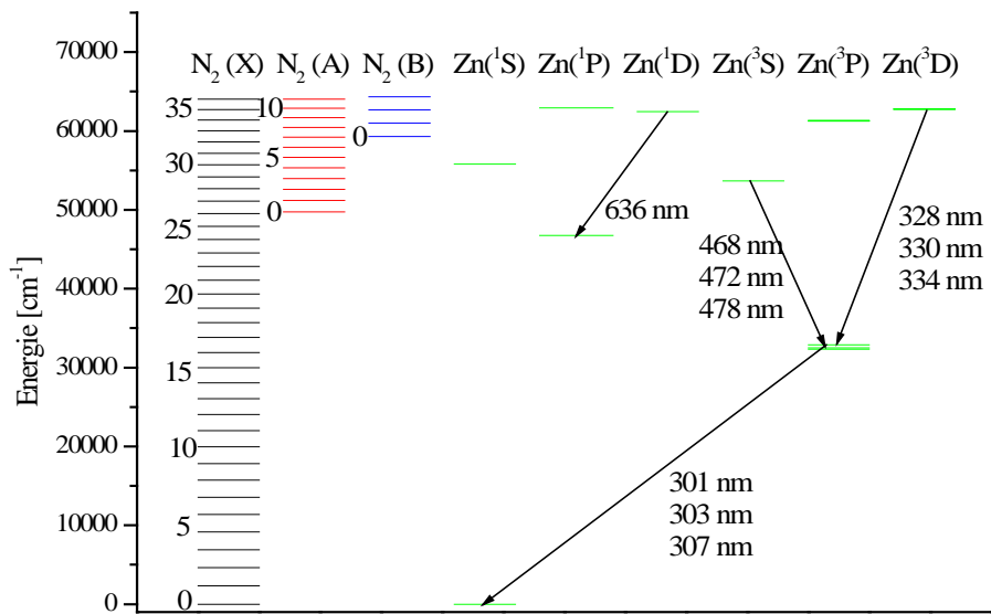
Obrázek 7: Energiové hladiny dusíku a zinku s vyznačenými vlnovými délkami spektrálních přechodů
