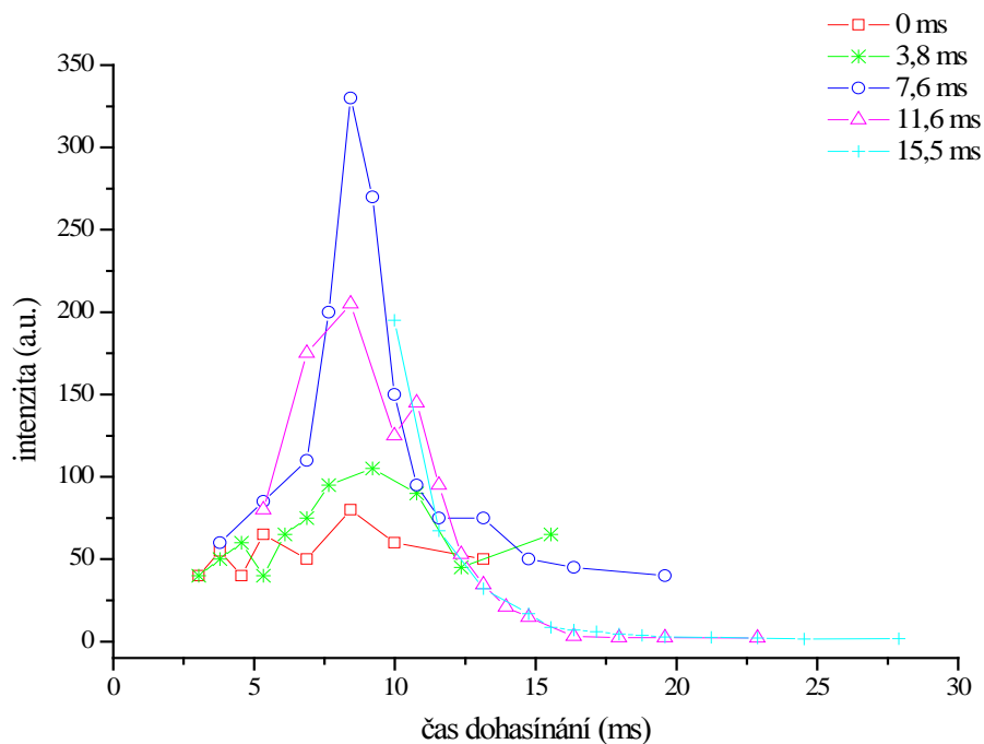
Obrázek 26: Závislost intenzity systému NO^\beta na čase dohasínání dusíkového plazmatu s příměsí rtuti
