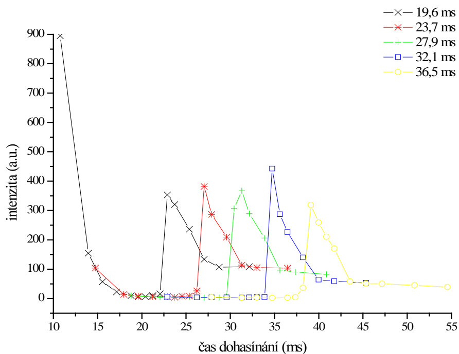
Obrázek 29: Závislost intenzity spektrální čáry rtuti na čase dohasinání dusíkového plazmatu s příměsí rtuti při různých vzdálenostech od aktivního výboje
