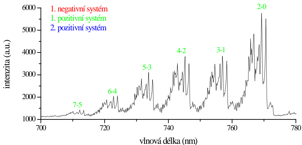
Obrázek 9: Ukázka identifikace optického emisního spektra dusíkového plazmatu (měřeno při tlaku 1050 Pa a čase dohasínání 20,6 ms)
