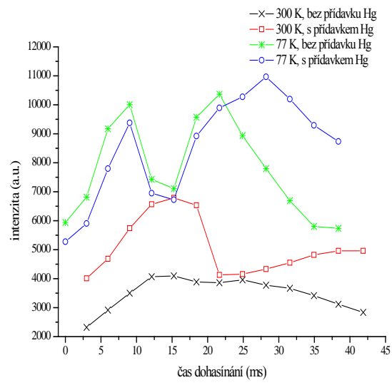
Obrázek 60: Průběh intenzity pásu 11-7 prvního pozitivního systému dusíku
