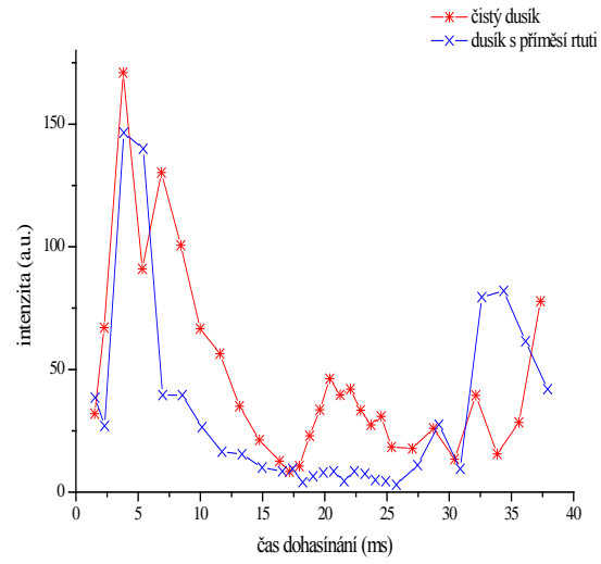
Obrázek 51: Průběh intenzity systému NO^{\beta}
