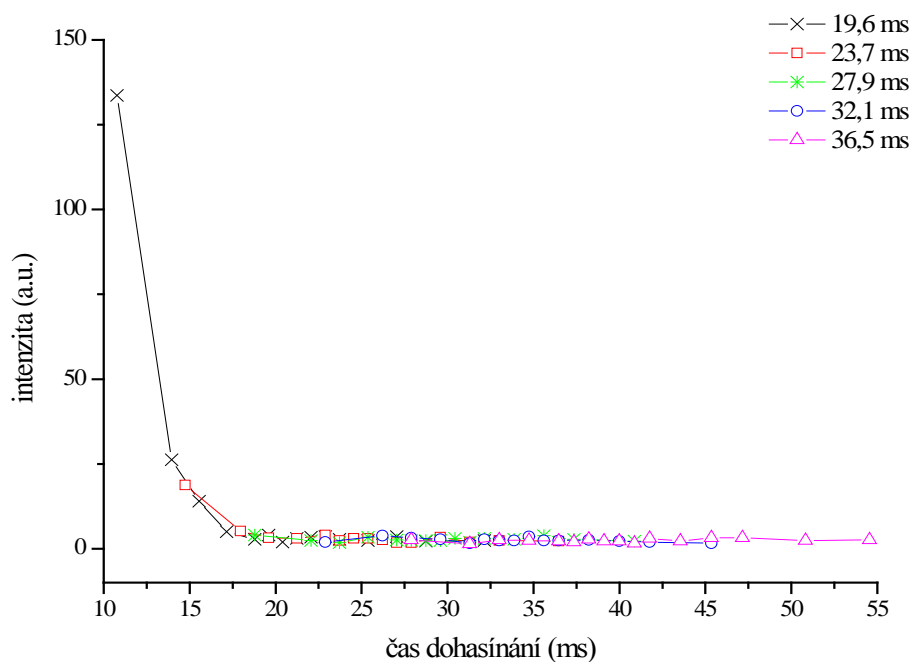
Obrázek 27: Závislost intenzity systému NO^\beta na čase dohasínání dusíkového plazmatu s příměsí rtuti
