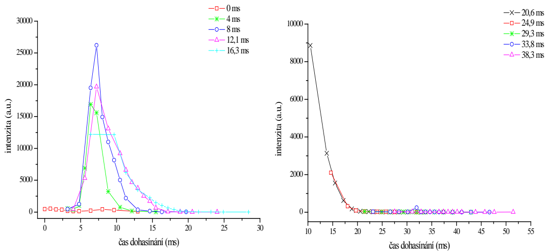
Obrázek 39: Závislost intenzity pásu 0-2 prvního negativního systému dusíku na čase dohasínání
