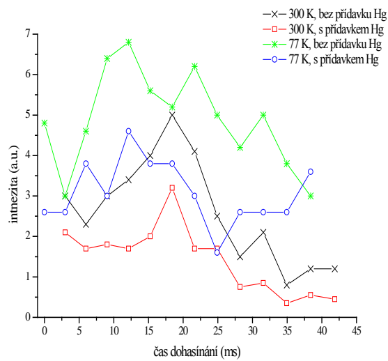
Obrázek 61: Průběh intenzity systému NO^\beta
