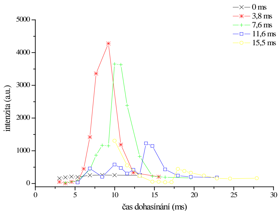
Obrázek 28: Závislost intenzity spektrální čáry rtuti na čase dohasinání dusíkového plazmatu s příměsí rtuti při různých vzdálenostech od aktivního výboje
