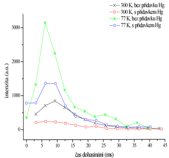
Obrázek 53: Průběh intenzity pásu 0-0 druhého pozitivního systému dusíku
