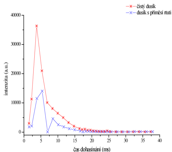
Obrázek 48: Průběh intenzity pásu 0-0 druhého pozitivního systému dusíku
