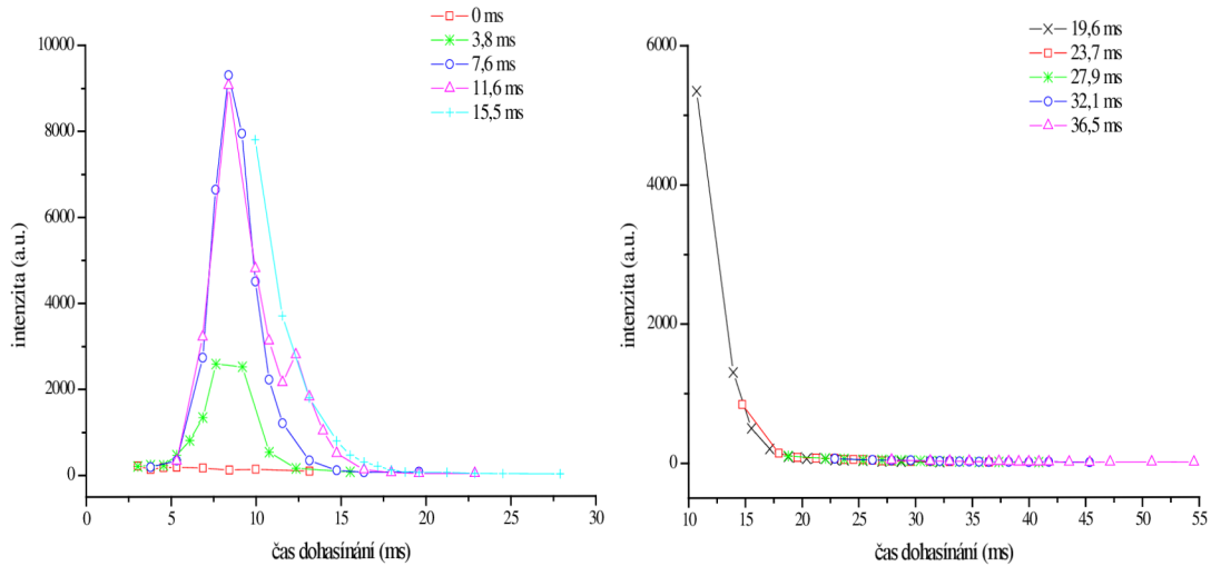
Obrázek 45: Závislost intenzity pásu 17-12 prvního pozitivního systému na čase dohasinání dusíkového plazmatu s příměsí rtuti
