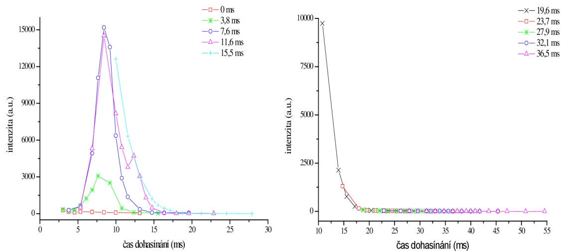
Obrázek 44: Závislost intenzity pásu 0-2 prvního negativního systému na čase dohasinání dusíkového plazmatu s příměsí rtuti
