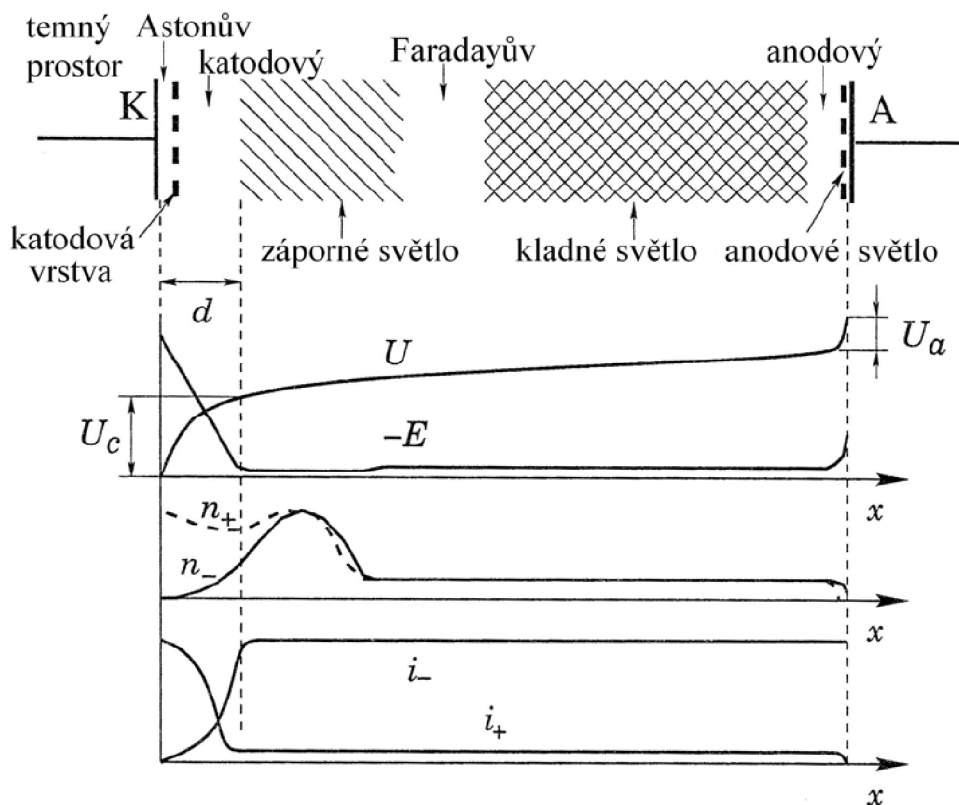
Obrázek 1: Struktura doutnavého výboje a průběhy podélného elektrického pole E , potenciálu U , koncentrace nabitých částic n^+ a n^- a hustoty proudů kladných iontů a elektronů i^+ a i^- [7]
