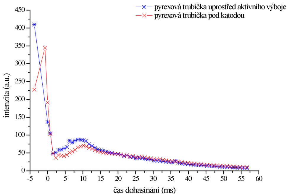
Obrázek 19: Závislost intenzity spektrální čáry rtuti na čase dohasinání dusíkového plazmatu s příměsí rtuti s pyrexovou trubičkou umístěnou uprostřed aktivního výboje a pod katodou
