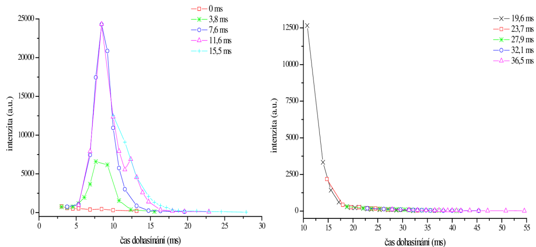
Obrázek 43: Závislost intenzity pásu 0-0 druhého pozitivního systému na čase dohasinání dusíkového plazmatu s příměsí rtuti
