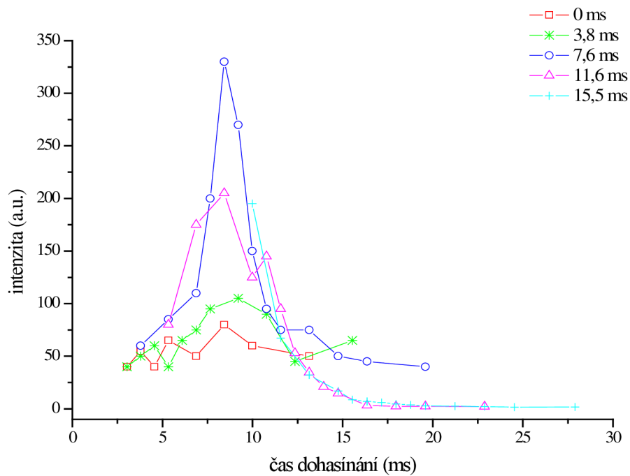
Obrázek 26: Závislost intenzity systému NO^\beta na čase dohasinání dusíkového plazmatu s příměsí rtuti
