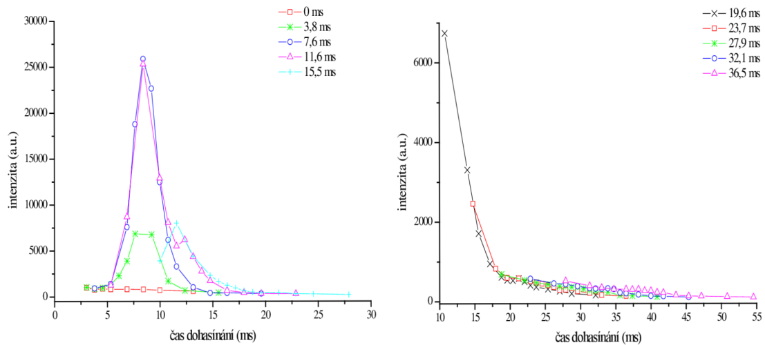
Obrázek 46: Závislost intenzity pásu 11-7 prvního pozitivního systému na čase dohasinání dusíkového plazmatu s příměsí rtuti
