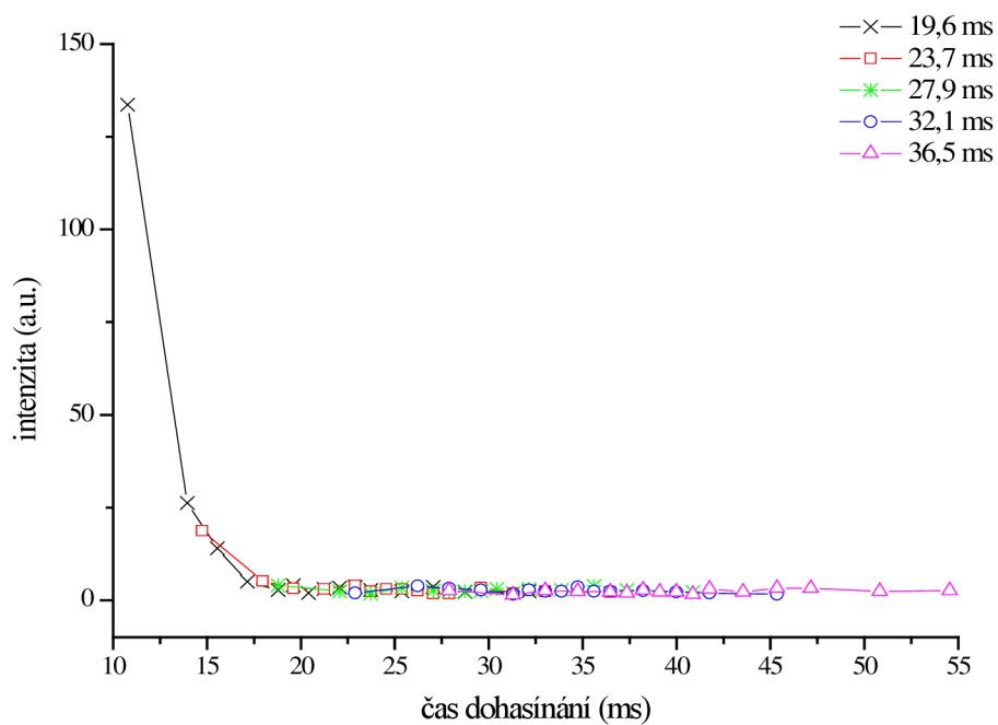
Obrázek 27: Závislost intenzity systému NO^\beta na čase dohasinání dusíkového plazmatu s příměsí rtuti
