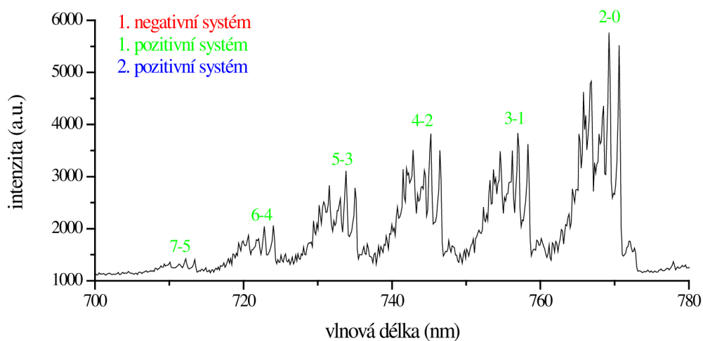
Obrázek 9: Ukázka identifikace optického emisního spektra dusíkového plazmatu (měřeno při tlaku 1050 Pa a čase dohasínání 20,6 ms)
